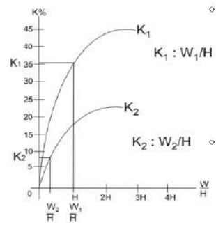
Figura 530.2.2 b. Curvas de coeficiente de Utilización
