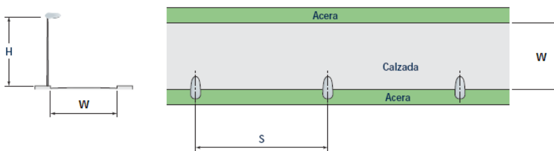
Figura 510.5.1 a. Disposición Unilateral
