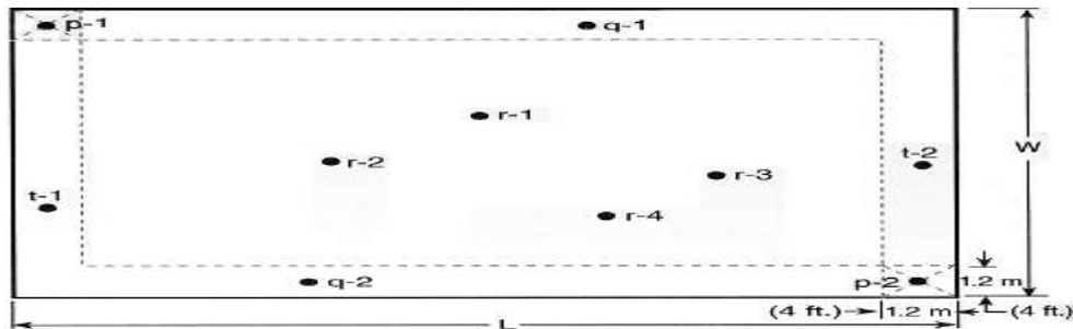
Figura 490.1 f) Puntos de medición de iluminancia en la cuadrícula de un local con cielorraso luminoso con luminarias con rejillas
