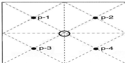
Figura 490.1 b. Puntos de medición de iluminancia de una luminaria en la cuadrícula de un local con una sola luminaria
