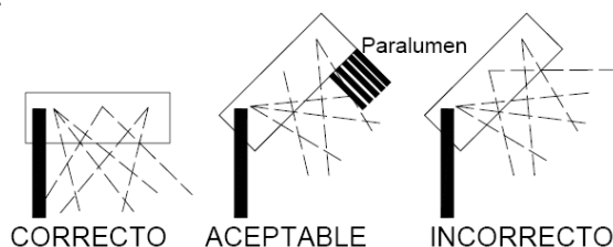
Figura 575.7.a) Control del flujo luminoso de proyectores
