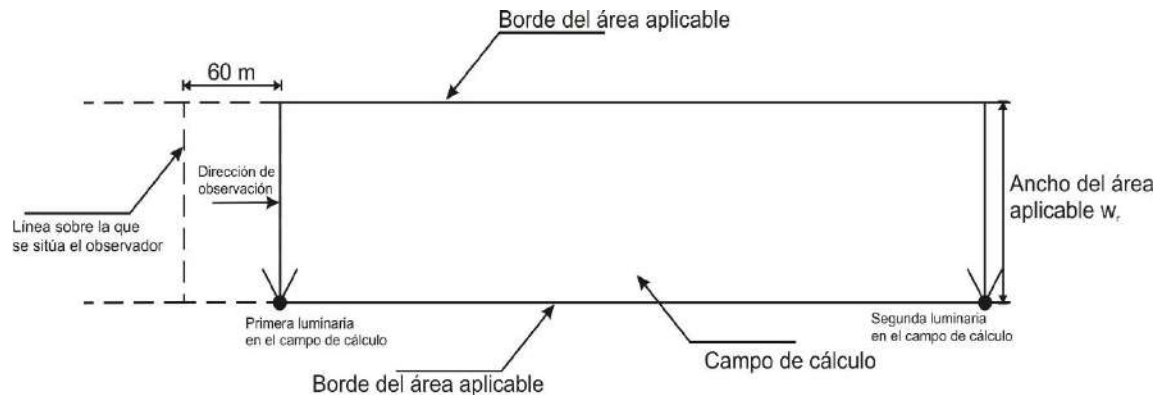
Figura 535.4 a. Campo de cálculo de la luminancia de la calzada
