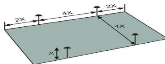
Figura 560.1 b. Ubicación de mástiles laterales al área
