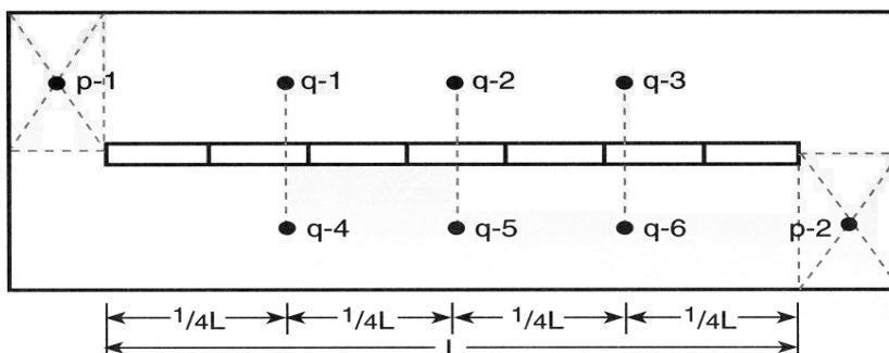
Figura 490.1 e. Puntos de medición de iluminancia en la cuadrícula de un local con una fila continua de luminarias
