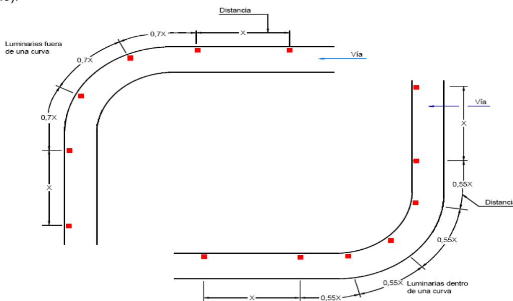
Figura 510.5.2 a. Disposición de luminarias en trayectos curvos
