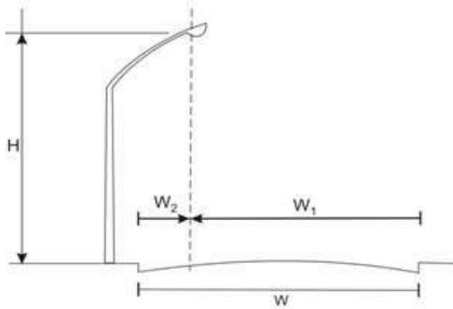
Figura 530.2.2 a. Determinación del Coeficiente de Utilización
