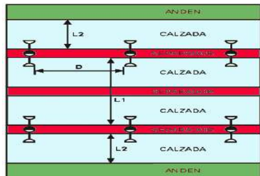
Figura 510.5.1 f. Disposición Doble central doble
