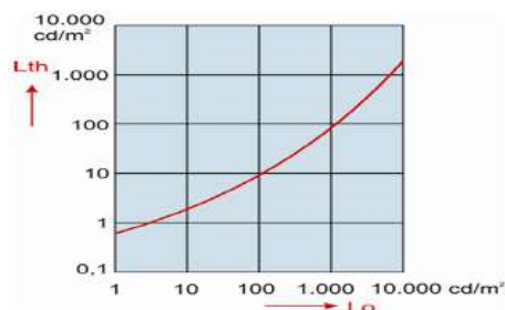
Figura 570.3 a. Nivel de iluminancia en túneles
