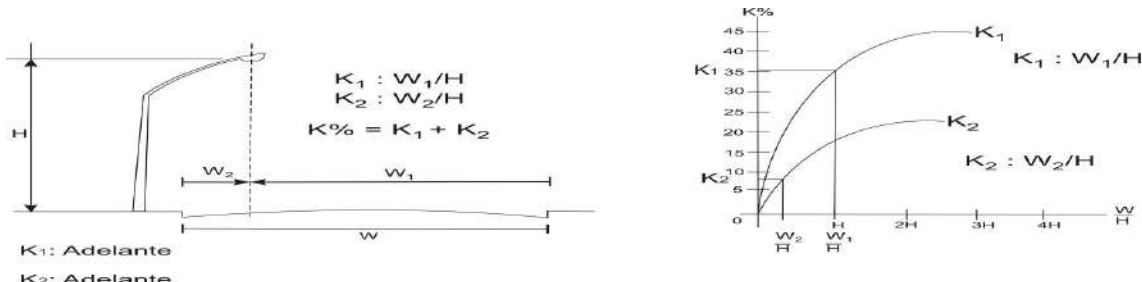
Figura 530.2.2 d. Luminaria sobre la calzada
