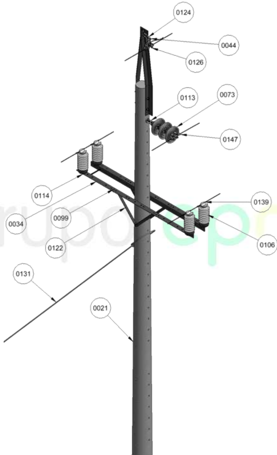
Figura 1. Vista isometrica.
