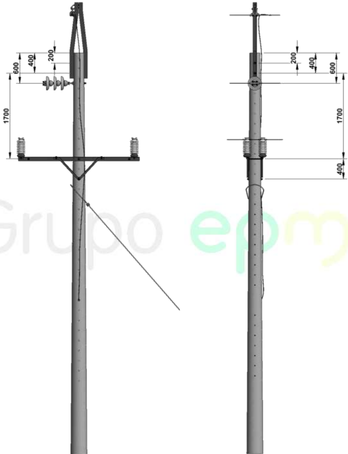
Figura 2. Vista frontal.
