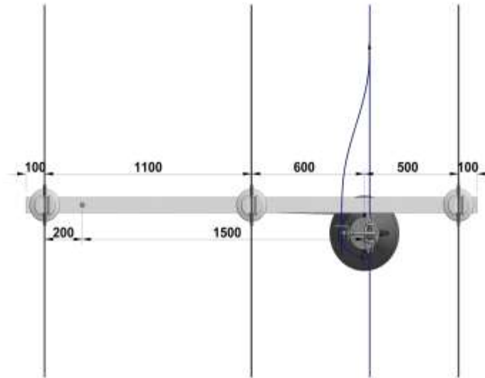
Figura 3. Vista en planta.
