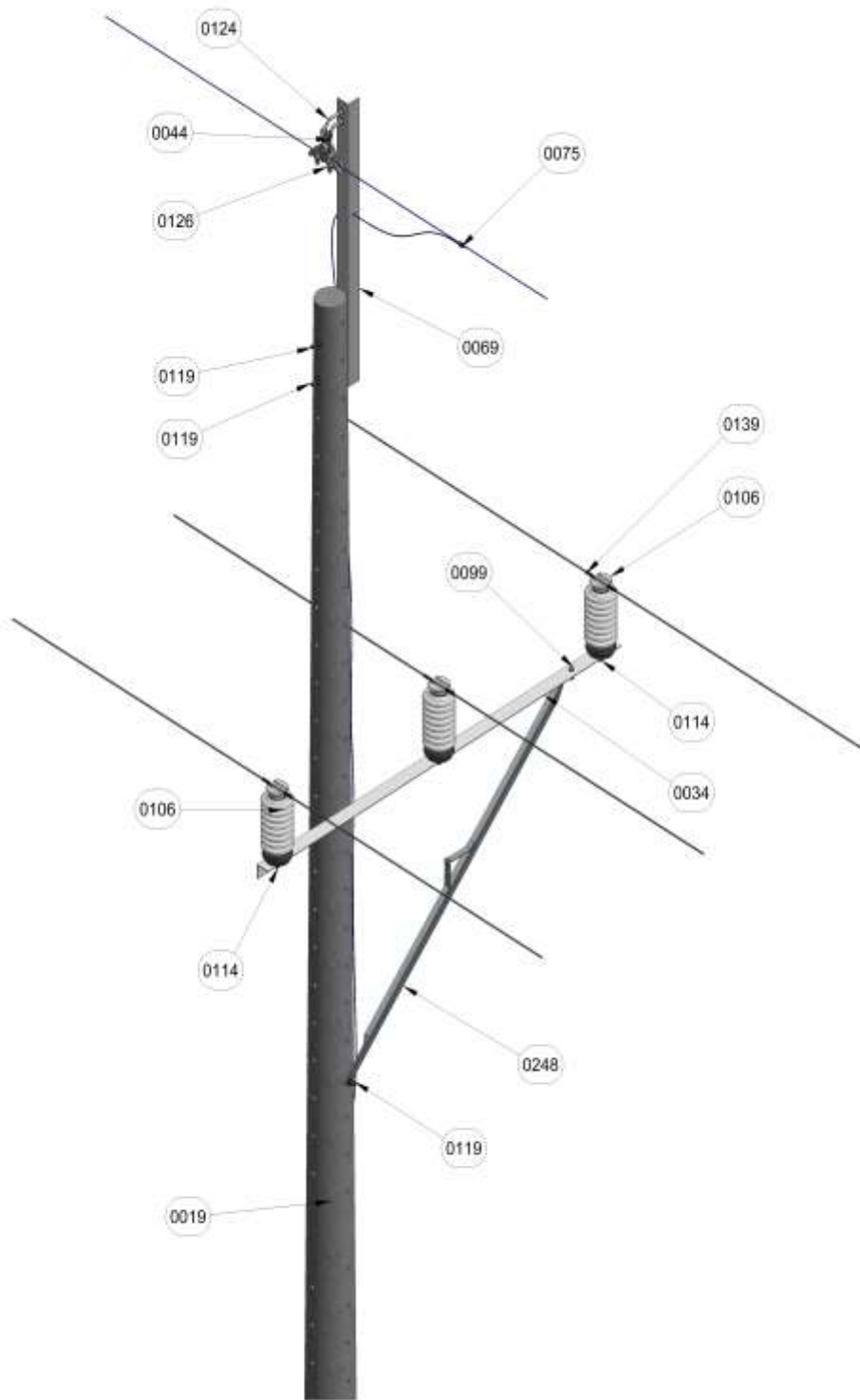
Figura 1. Vista isometrica.
