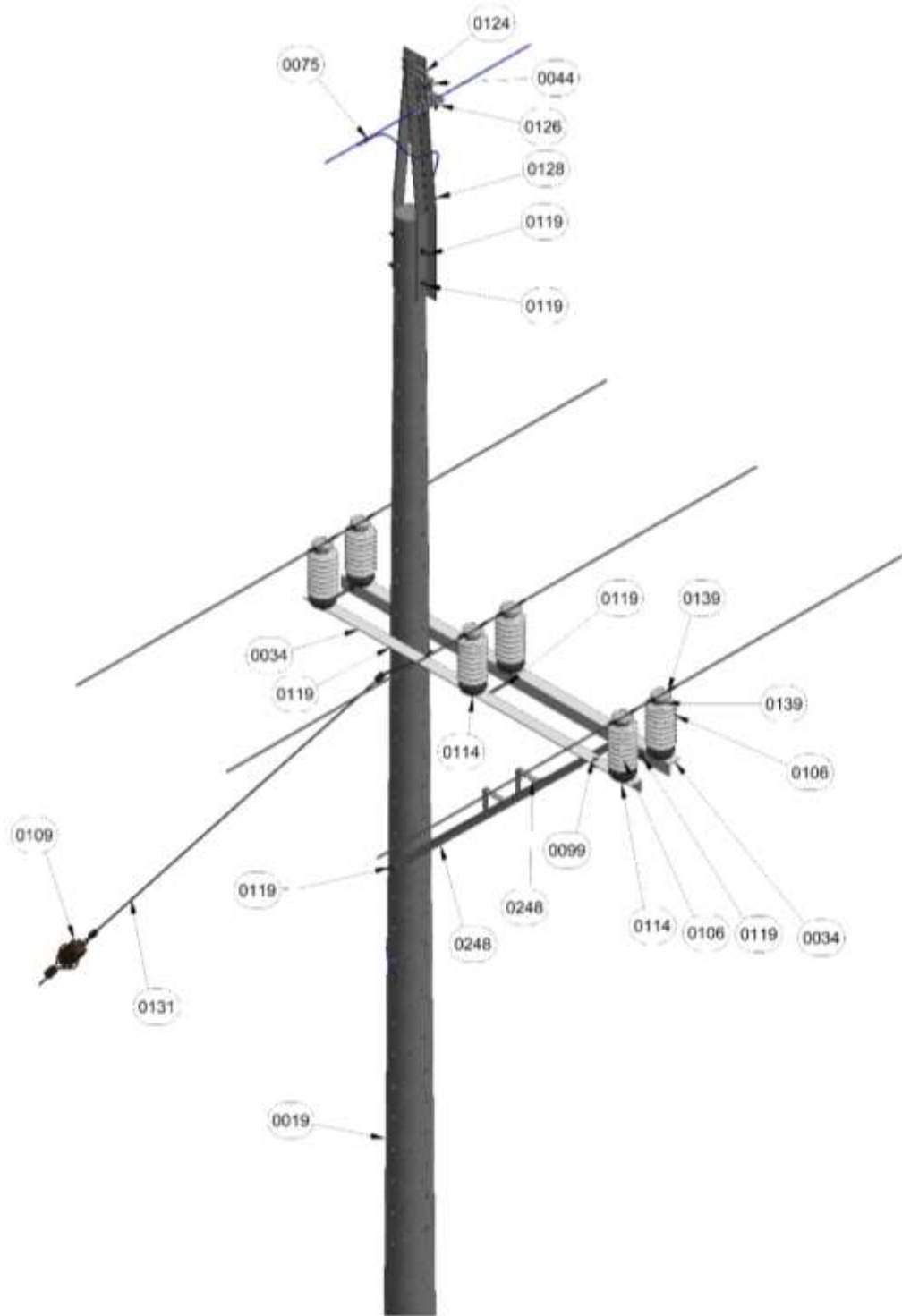
Figura 1. Vista isometrica.
