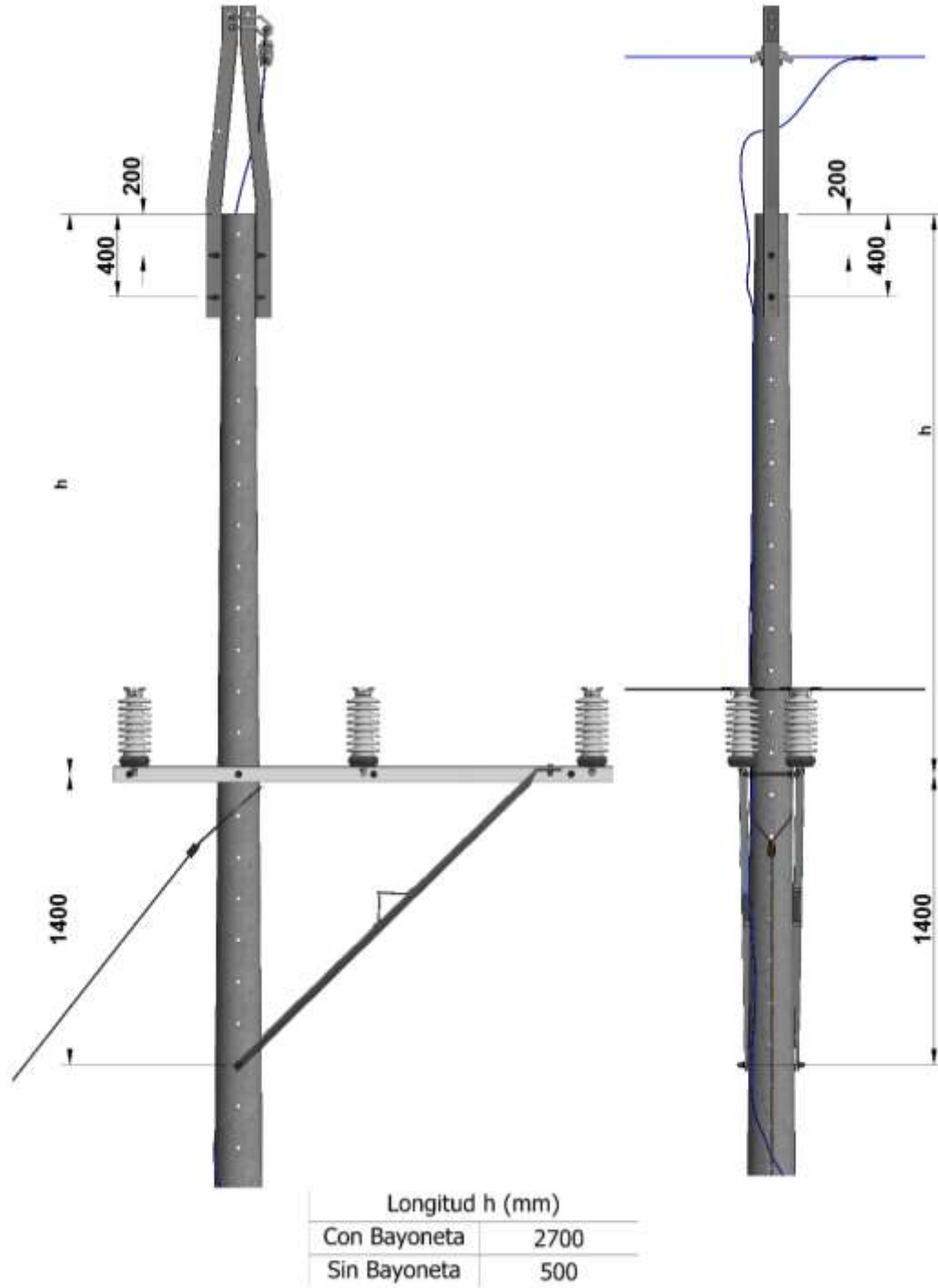
Figura 2. Vista frontal.
