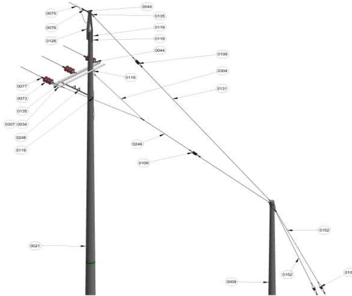
Figura 1. Vista isometrica.
