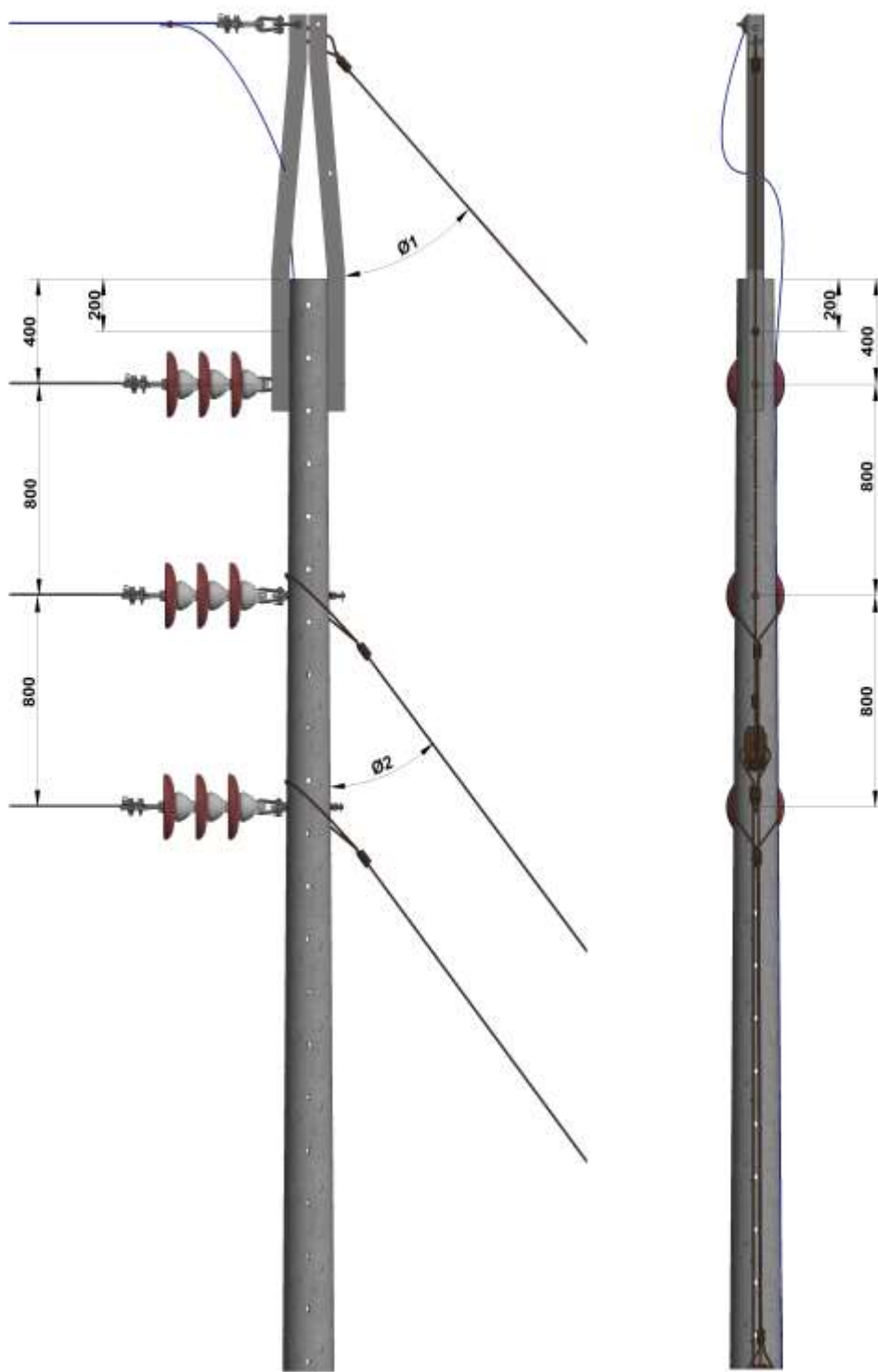
Figura 2. Vista frontal.
