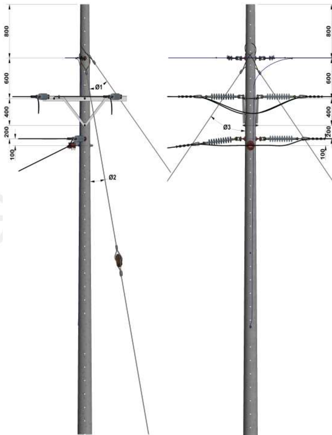
Figura 2. Vista frontal.
