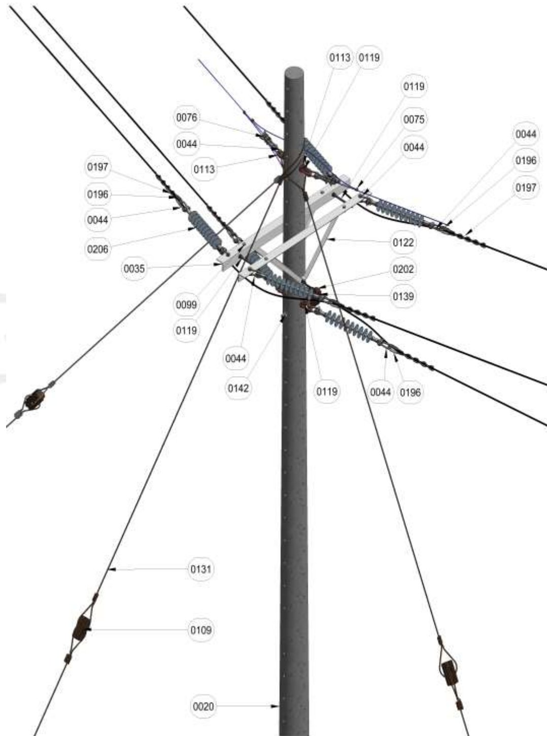
Figura 1. Vista isométrica.
