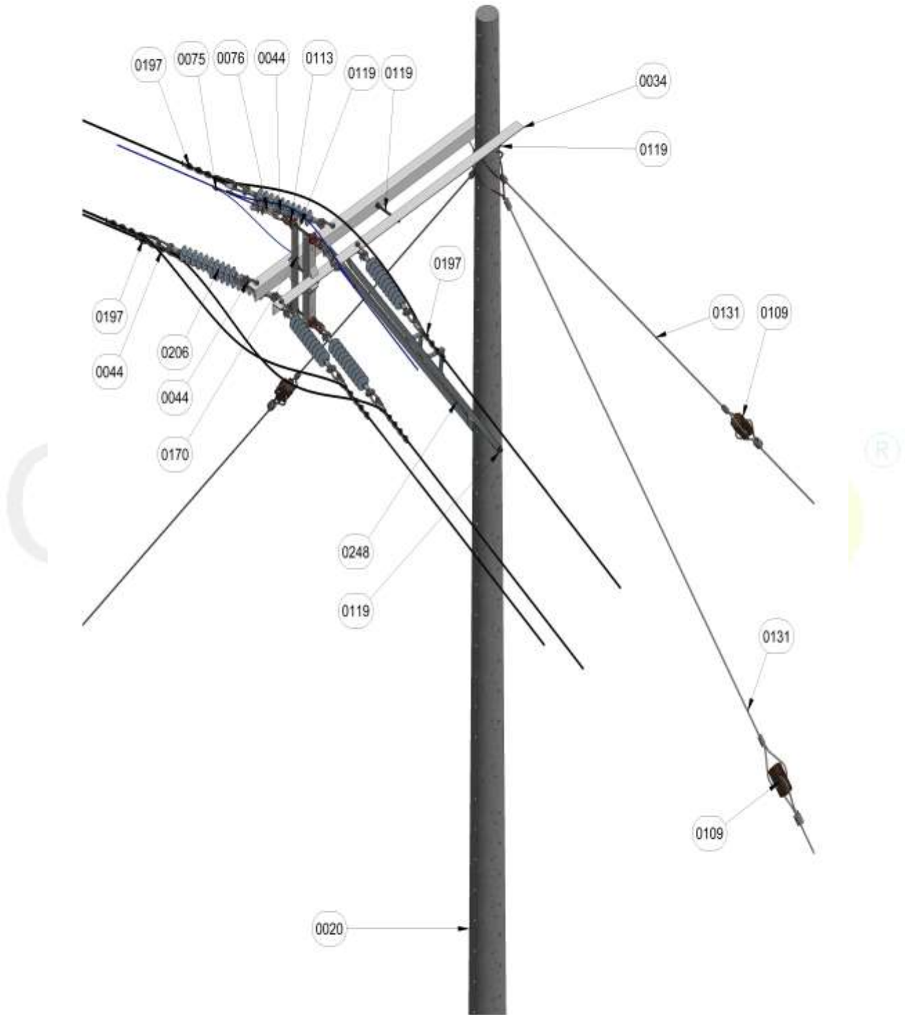
Figura 1. Vista isometrica.
