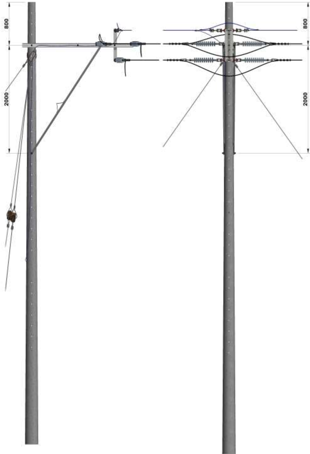
Figura 2. Vista frontal.
