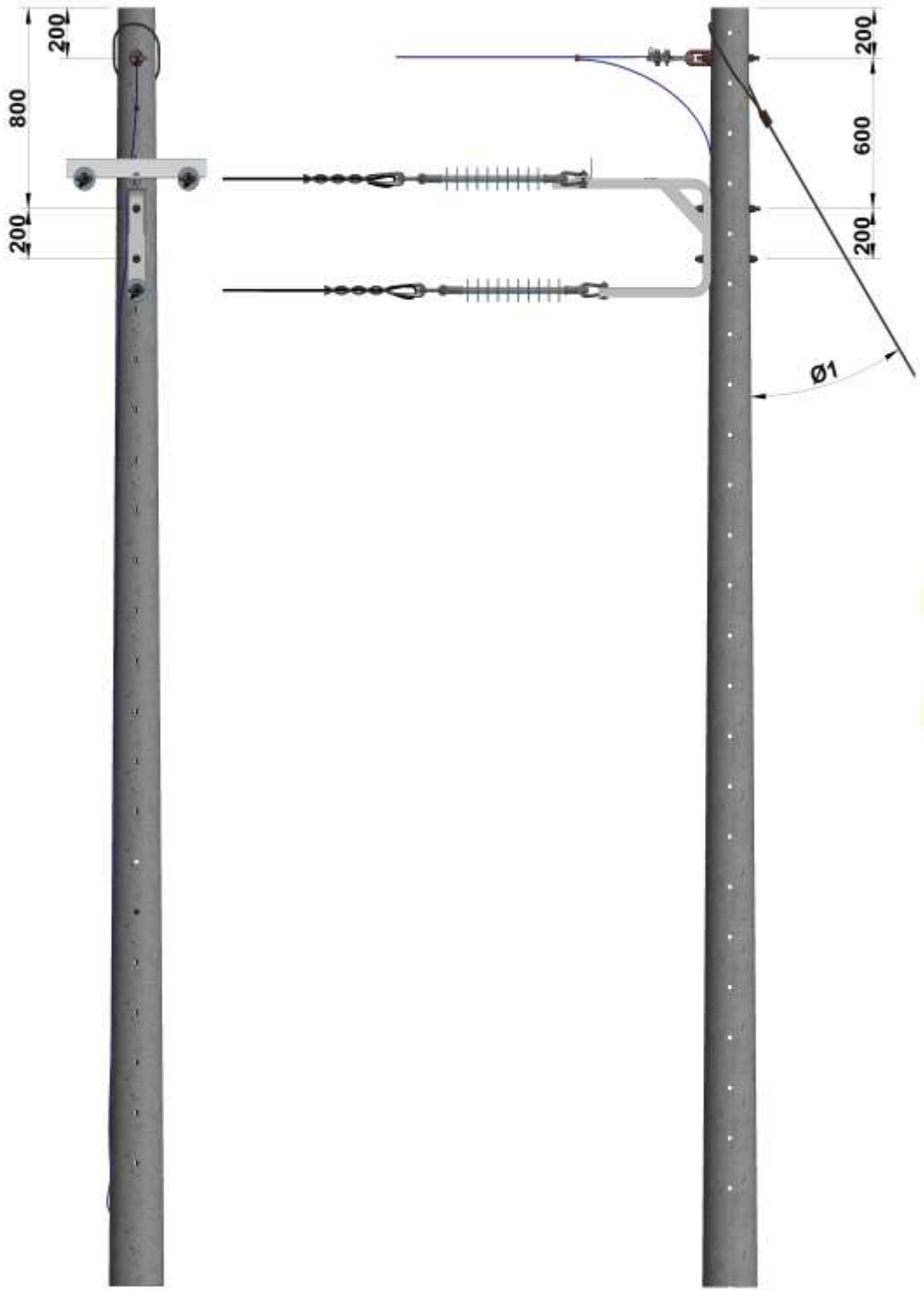
Figura 2. Vista frontal.
