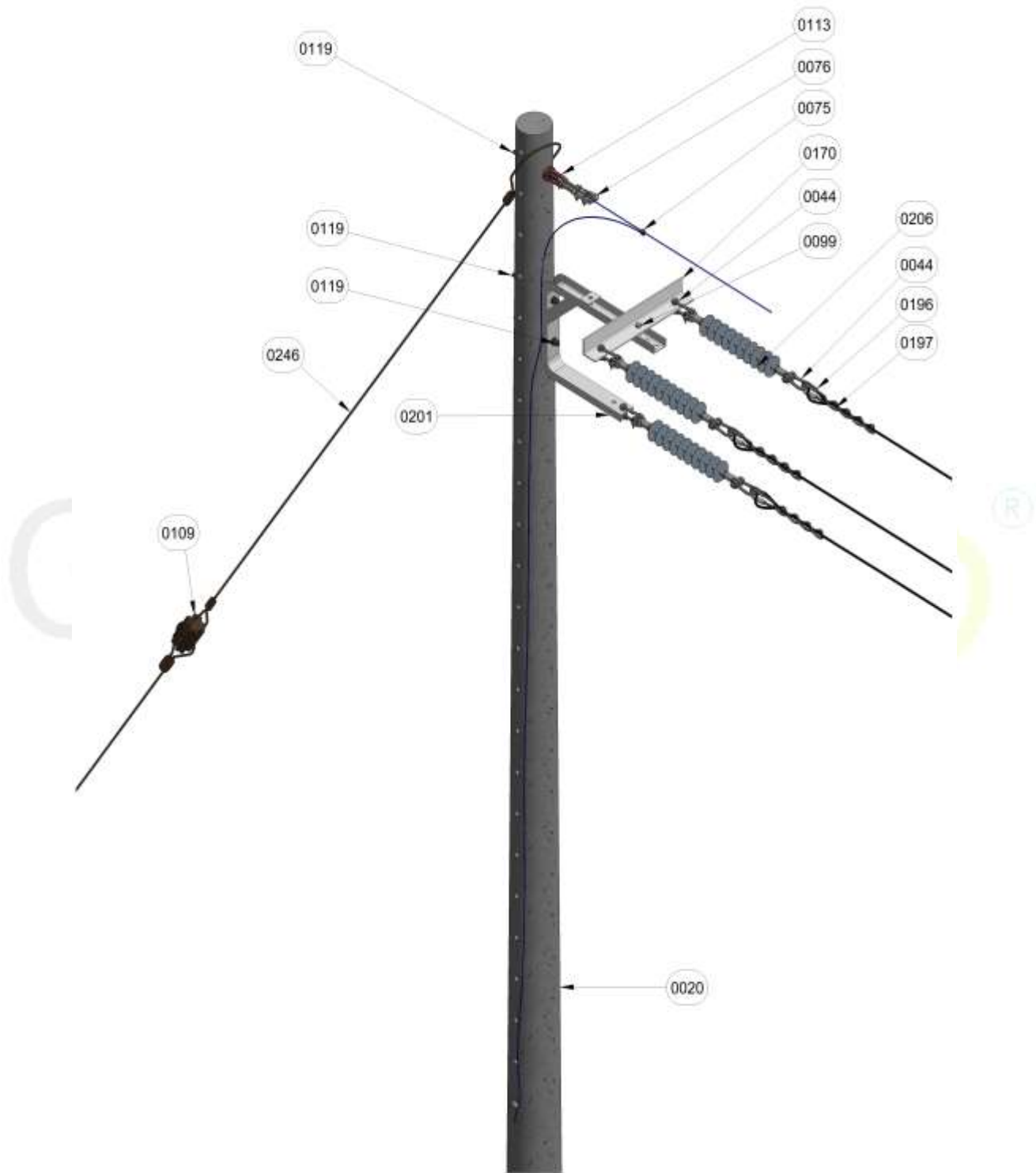
Figura 1. Vista isometrica.
