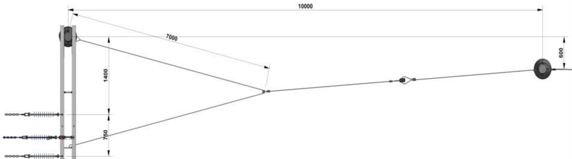
Figura 3. Vista en planta.
