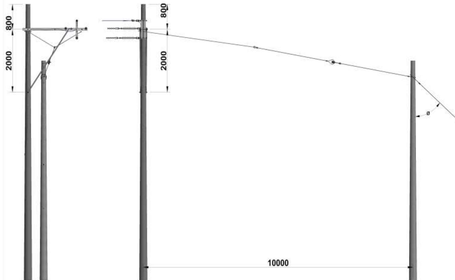
Figura 2. Vista frontal.
