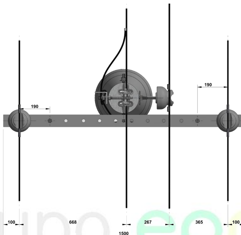
Figura 3. Vista en planta
