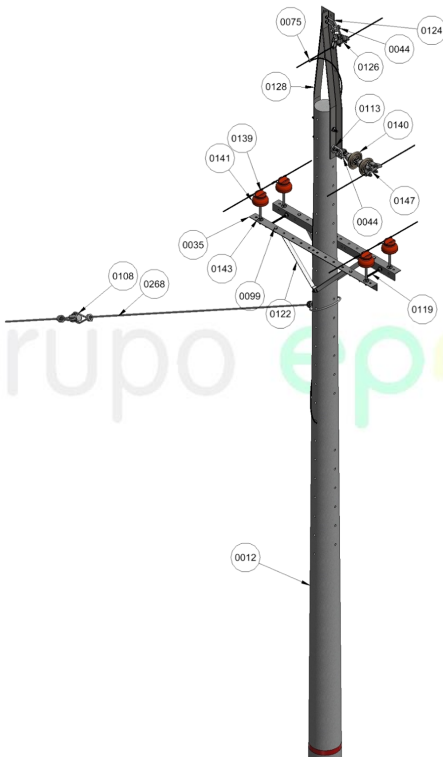
Figura 1. Vista isometrica
