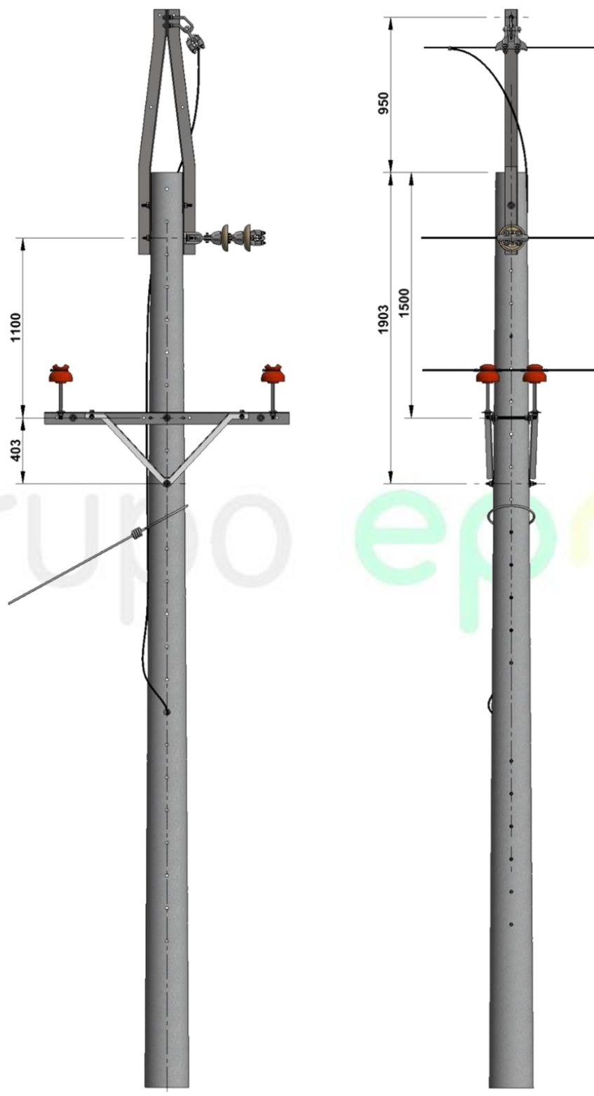
Figura 2. Vista frontal
