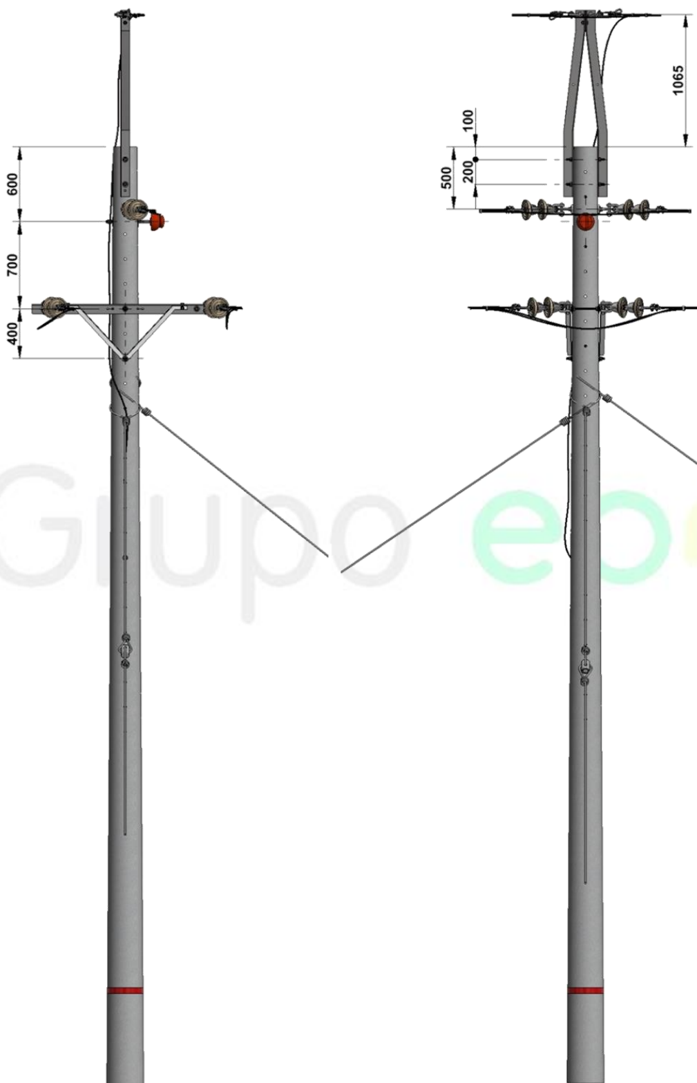
Figura 2. Vista frontal
