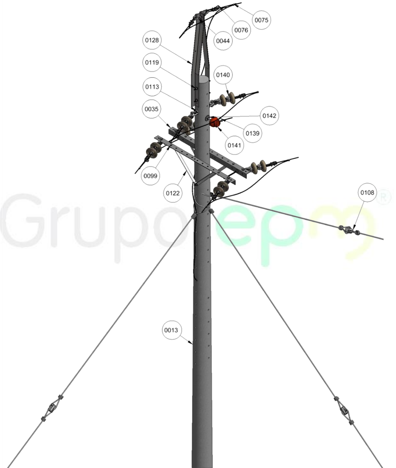
Figura 1. Vista isometrica
