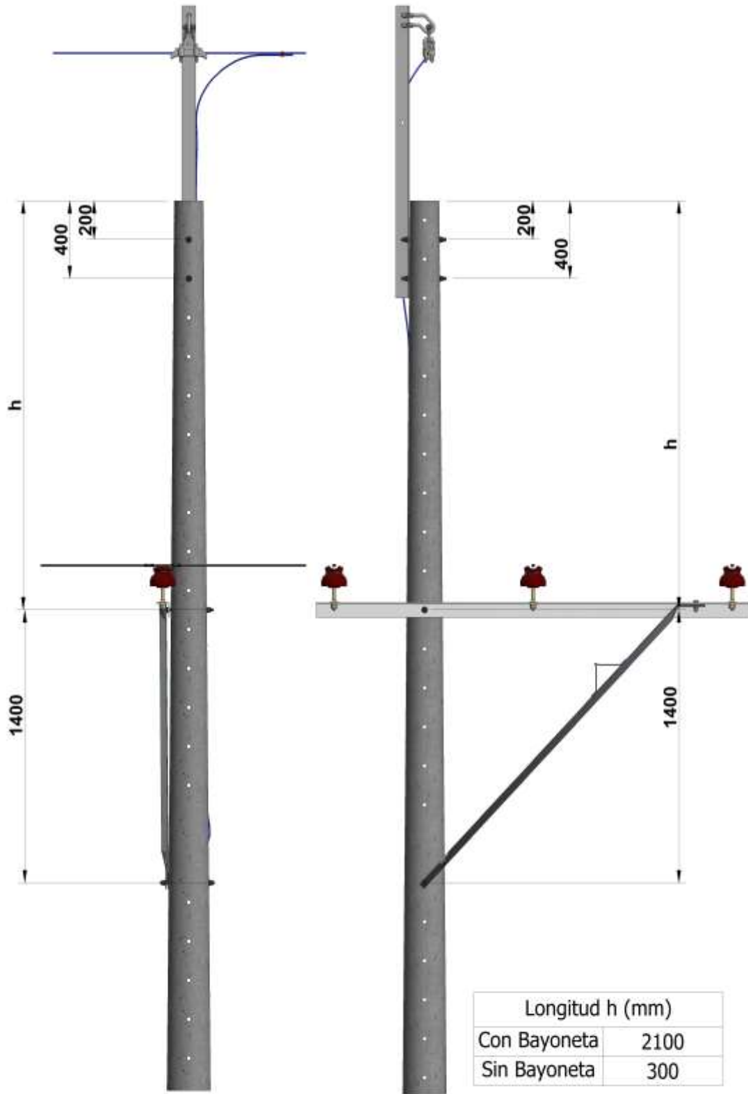
Figura 2. Vista frontal
