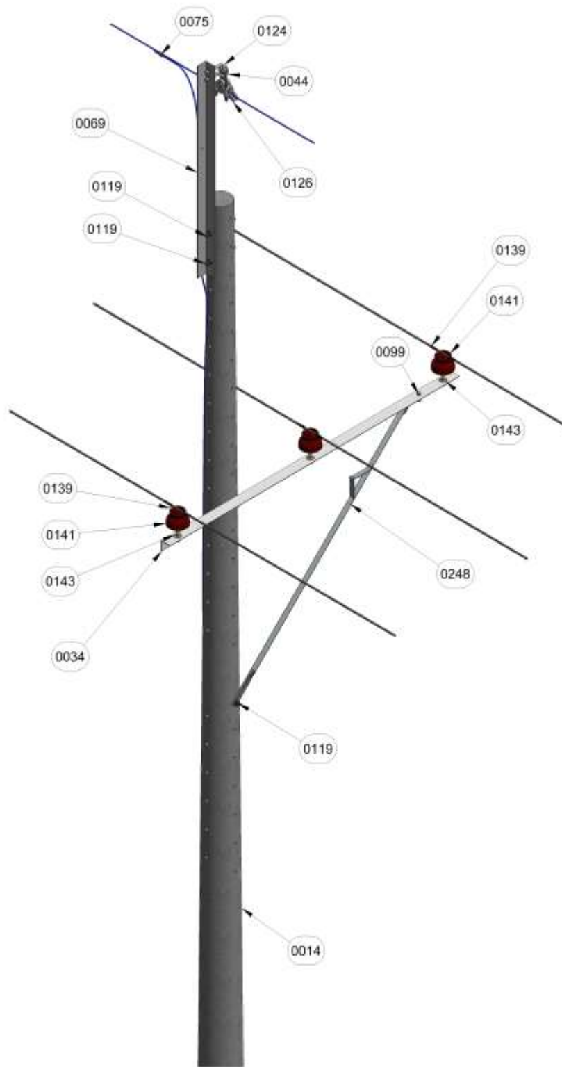
Figura 1. Vista isométrica
