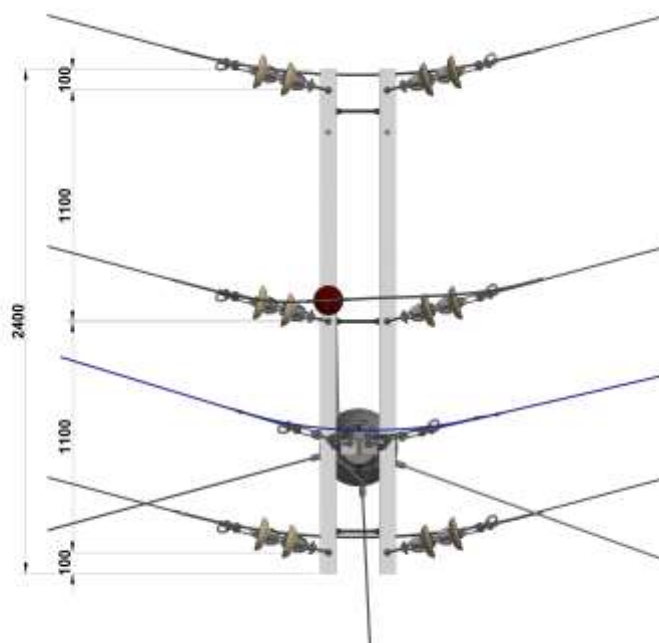
Figura 3. Vista en planta
