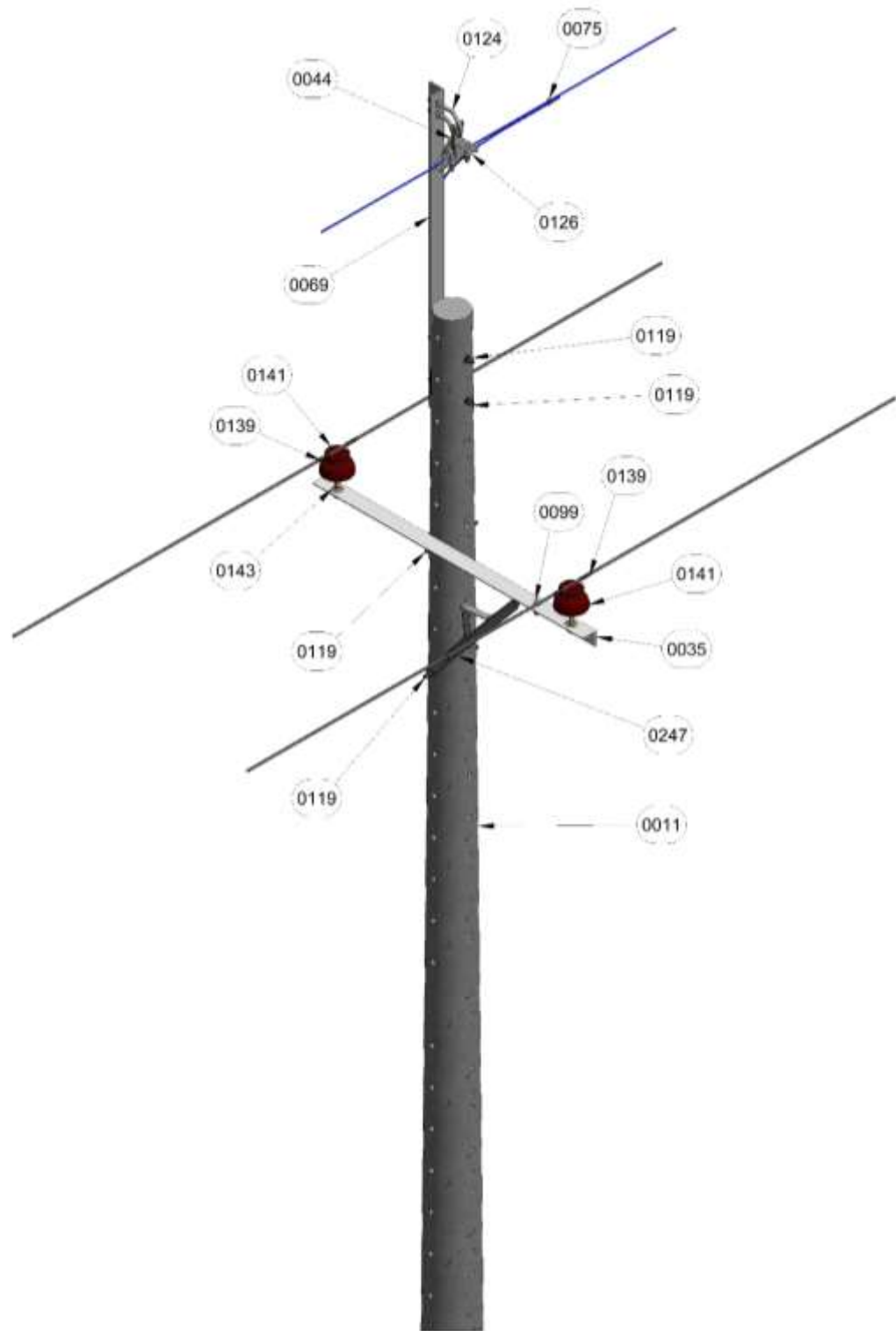
Figura 1. Vista isometrica
