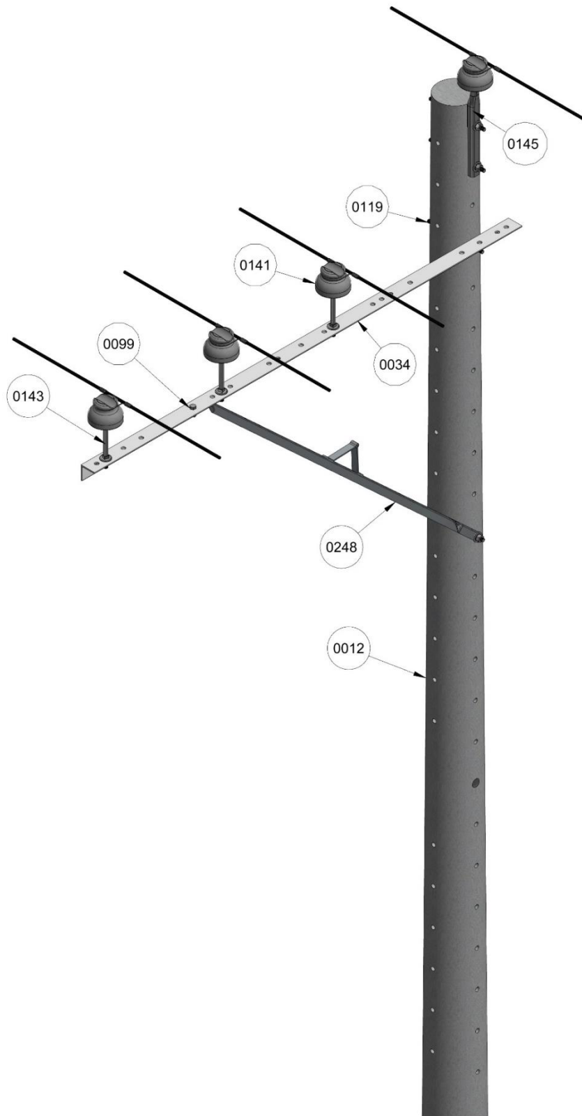
Figura 1. Vista isometrica.
