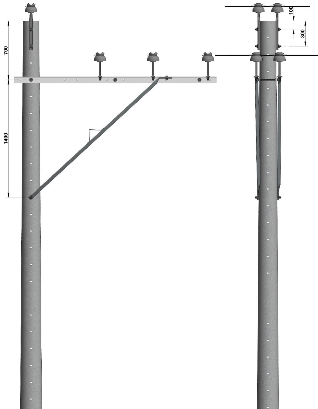
Figura 2. Vista frontal.
