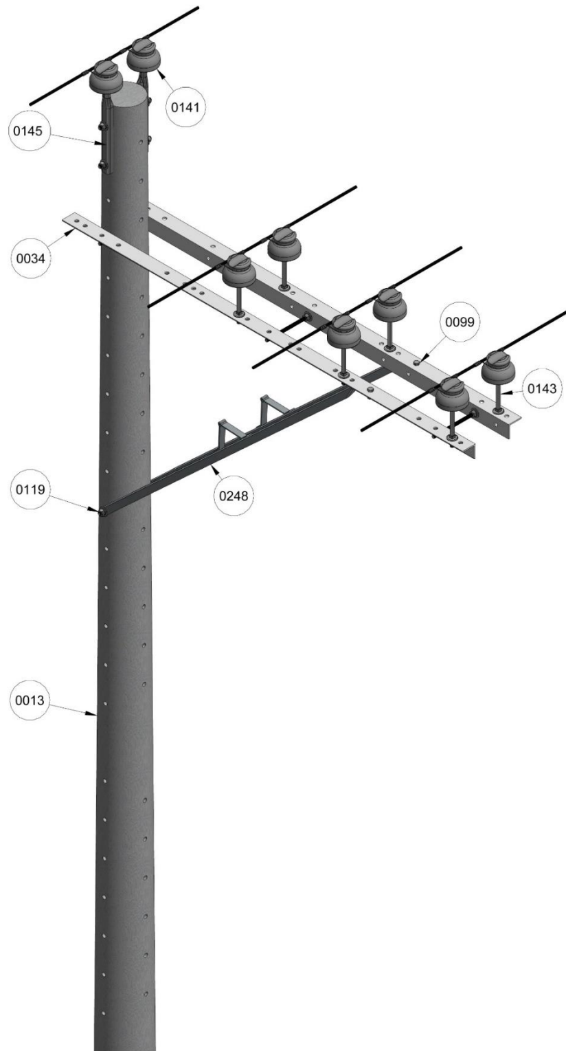
Figura 1. Vista isometrica.
