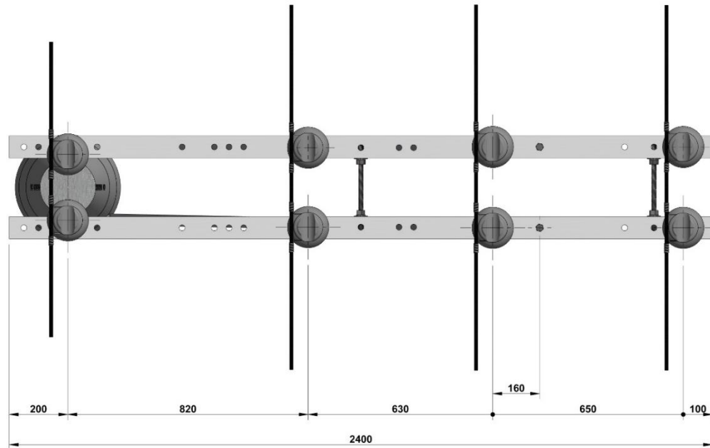
Figura 3. Vista en planta.
