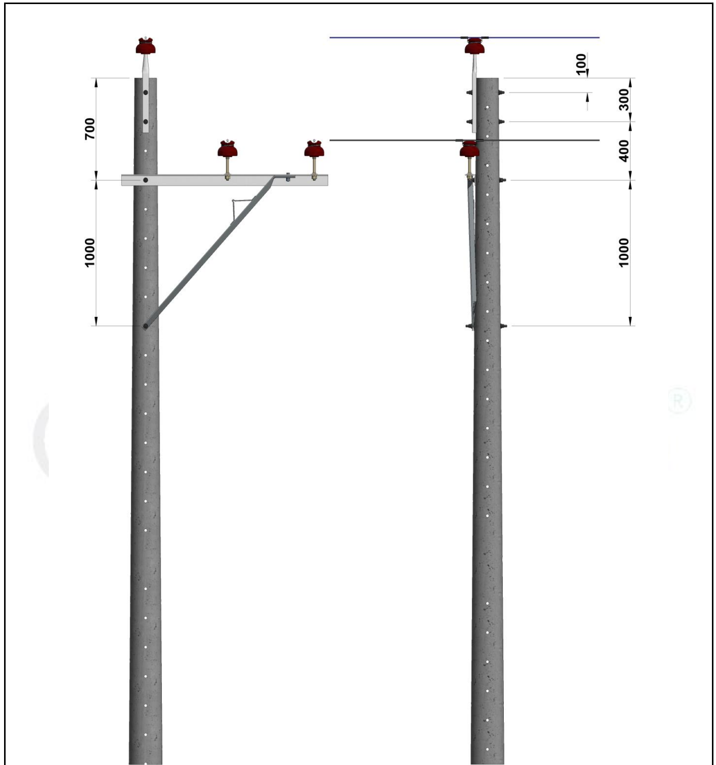
Figura 2. Vista frontal.
