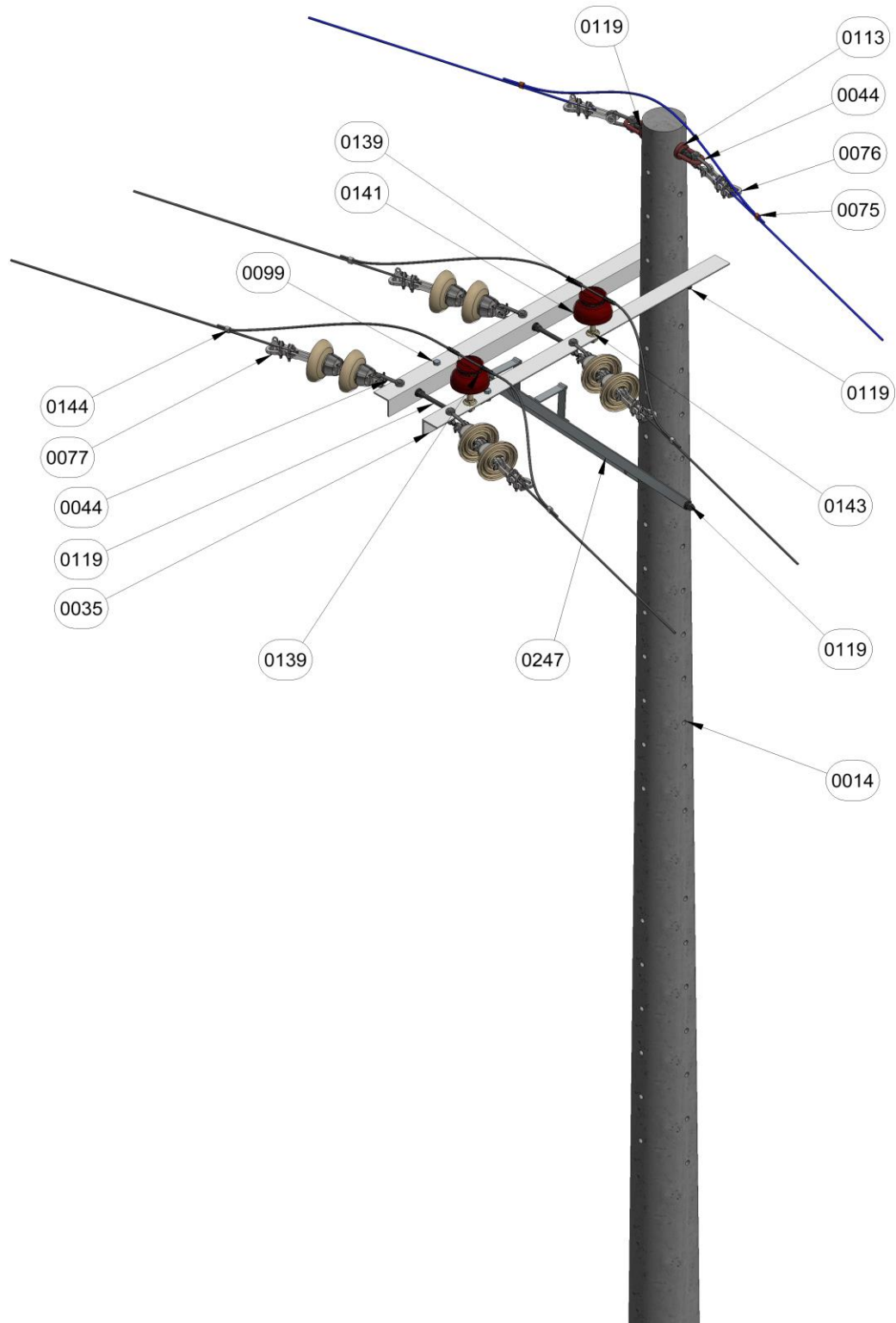
Figura 1. Vista isometrica.
