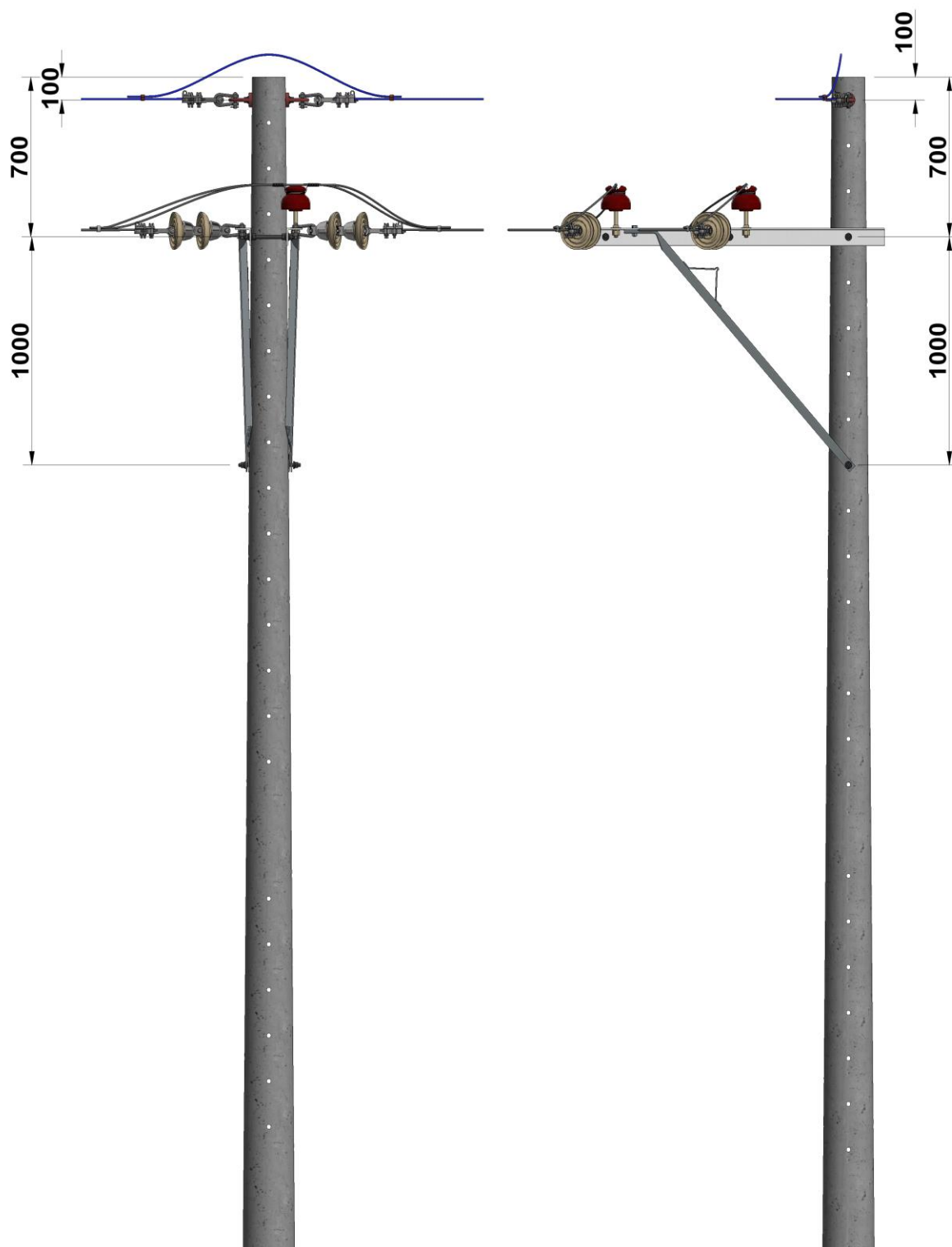
Figura 2. Vista frontal.
