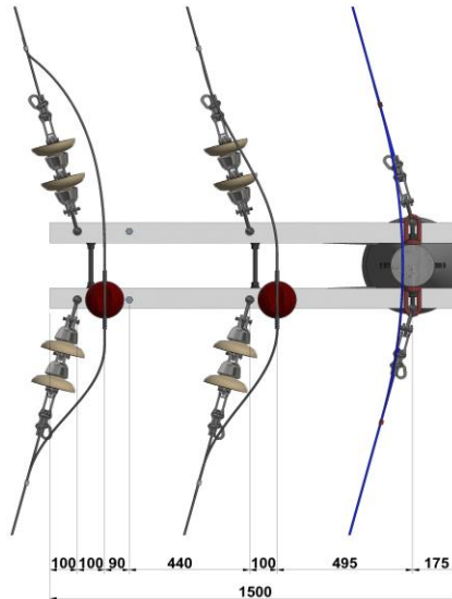
Figura 3. Vista en planta.
