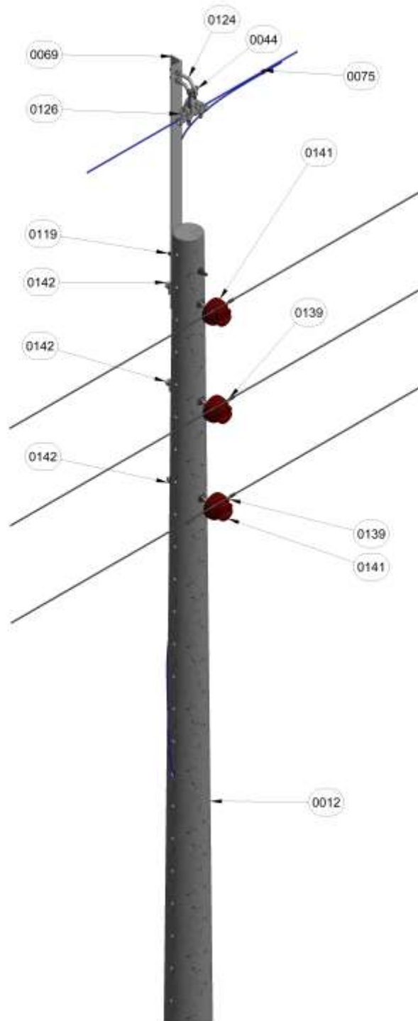
Figura 1. Vista isometrica.
