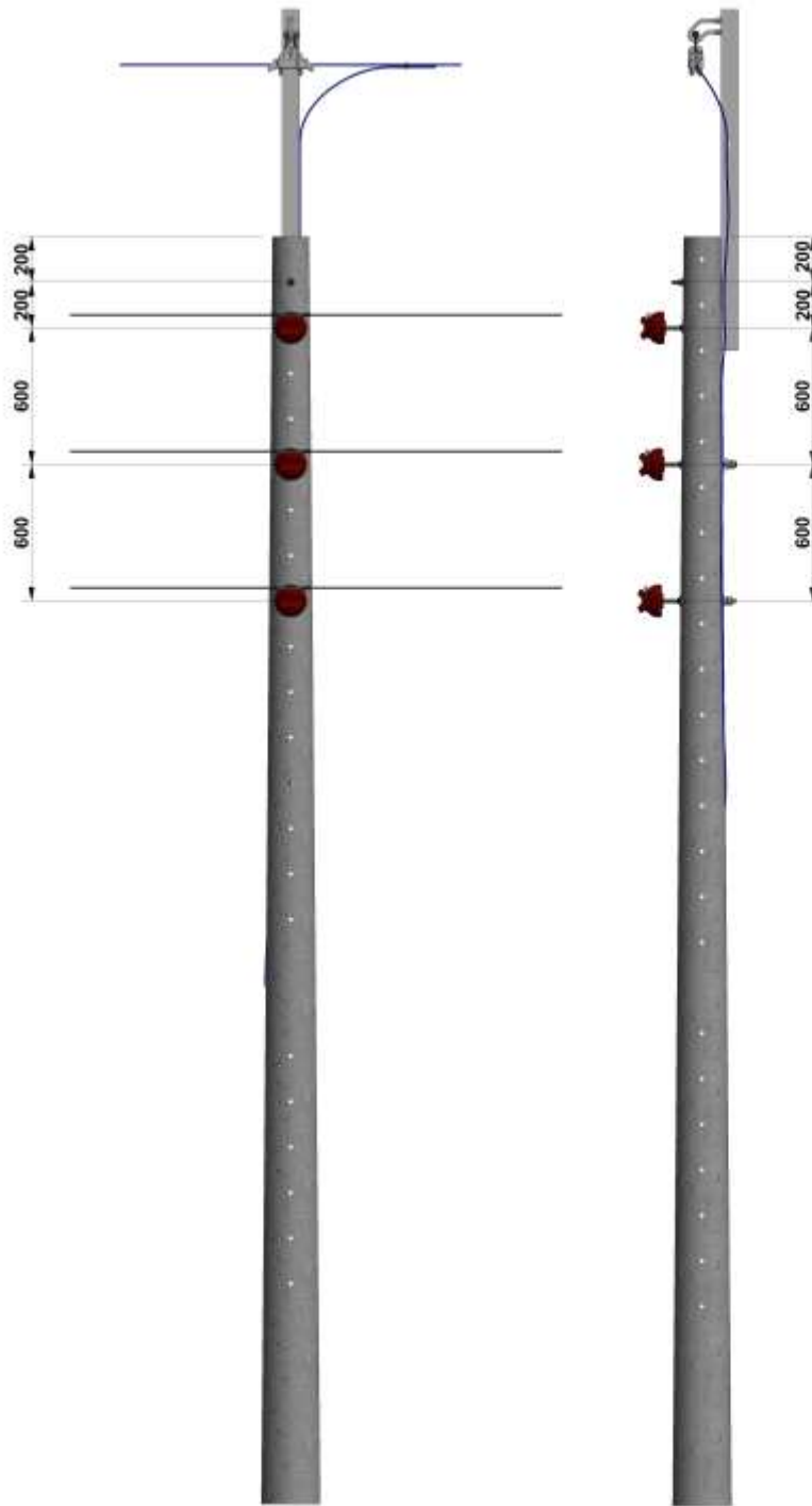
Figura 2. Vista frontal.
