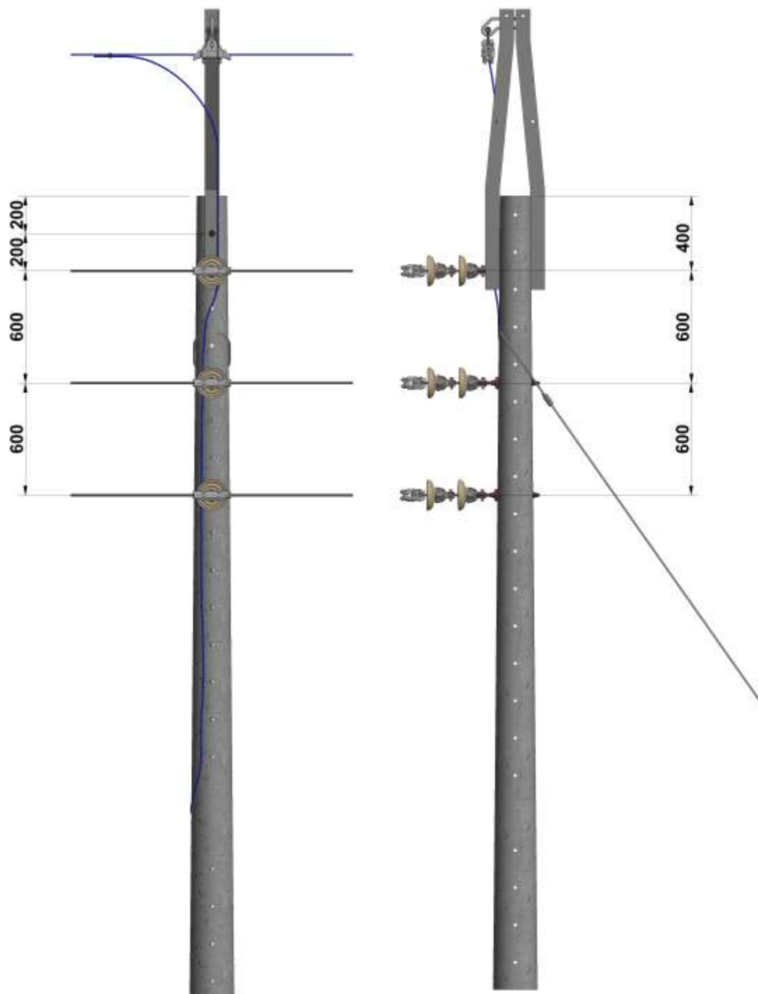
Figura 2. Vista frontal.
