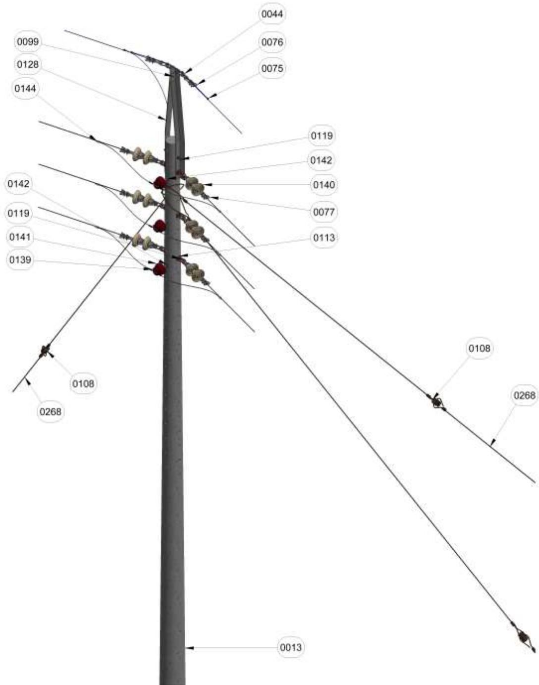
Figura 1. Vista isometrica.
