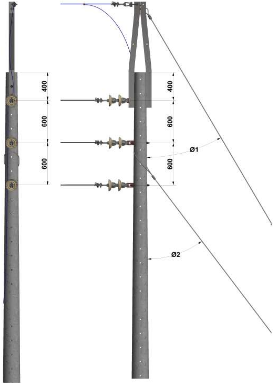
Figura 2. Vista frontal.
