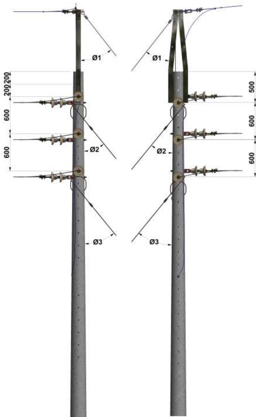
Figura 2. Vista frontal.
