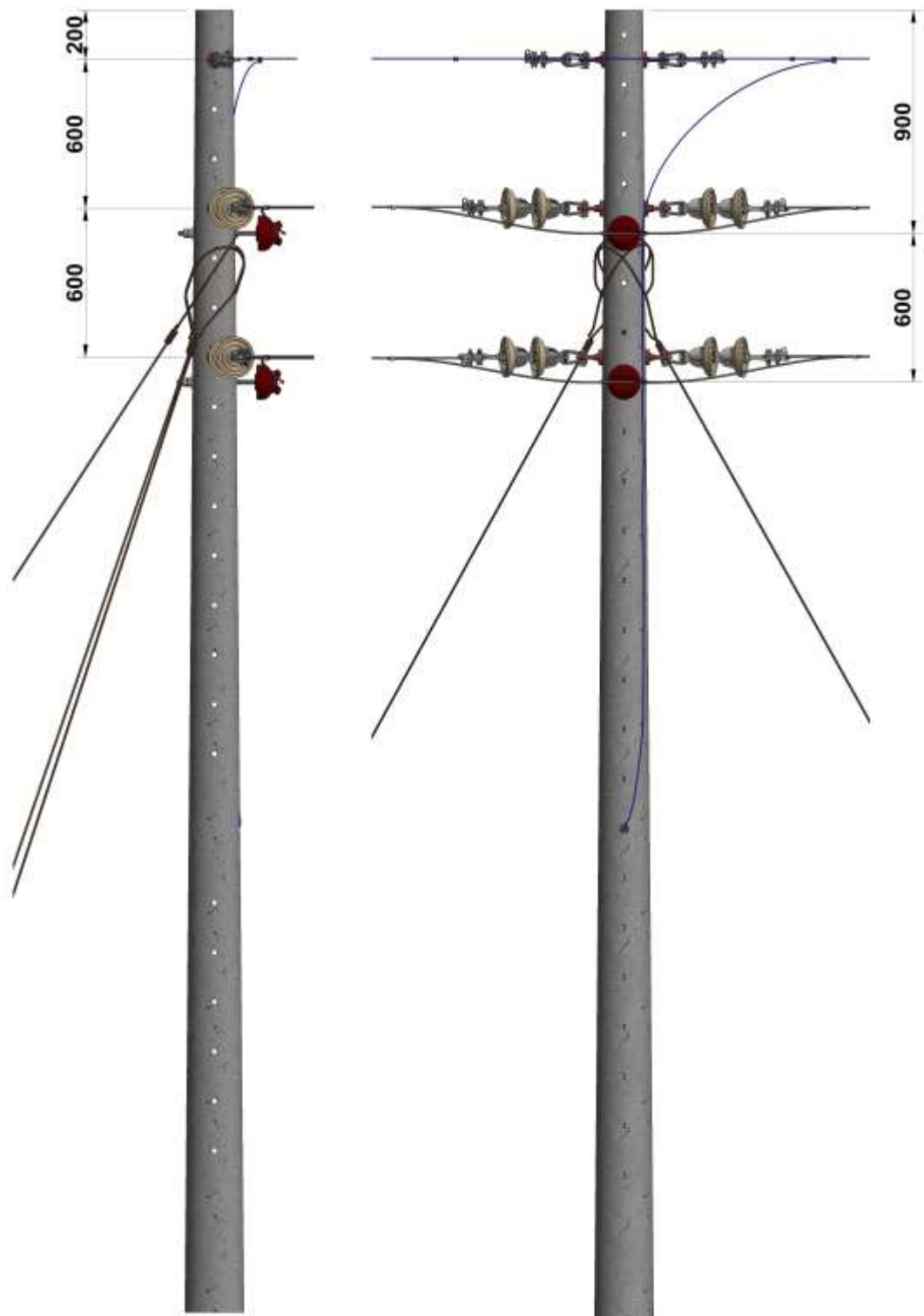
Figura 2. Vista frontal.
