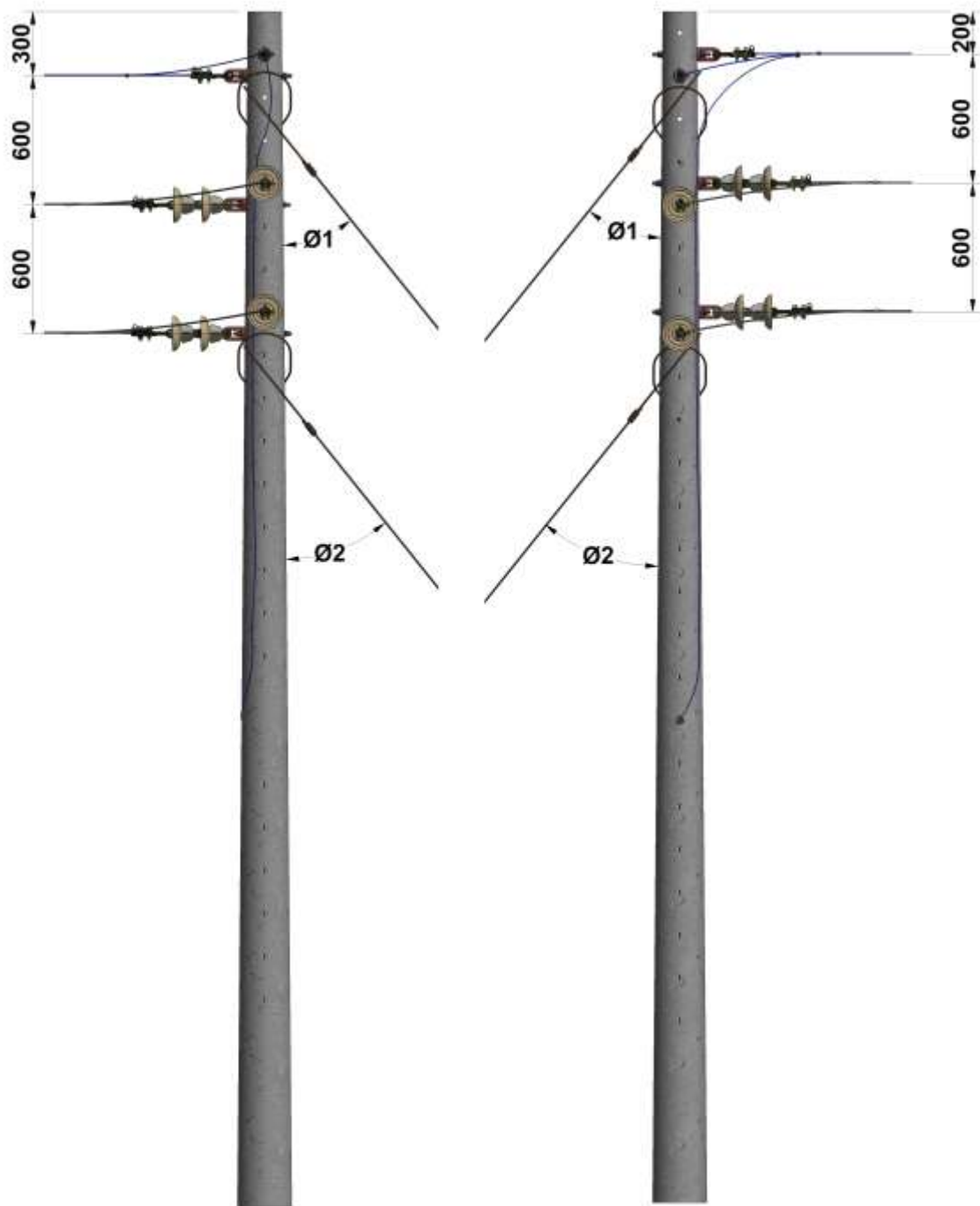
Figura 2. Vista frontal.
