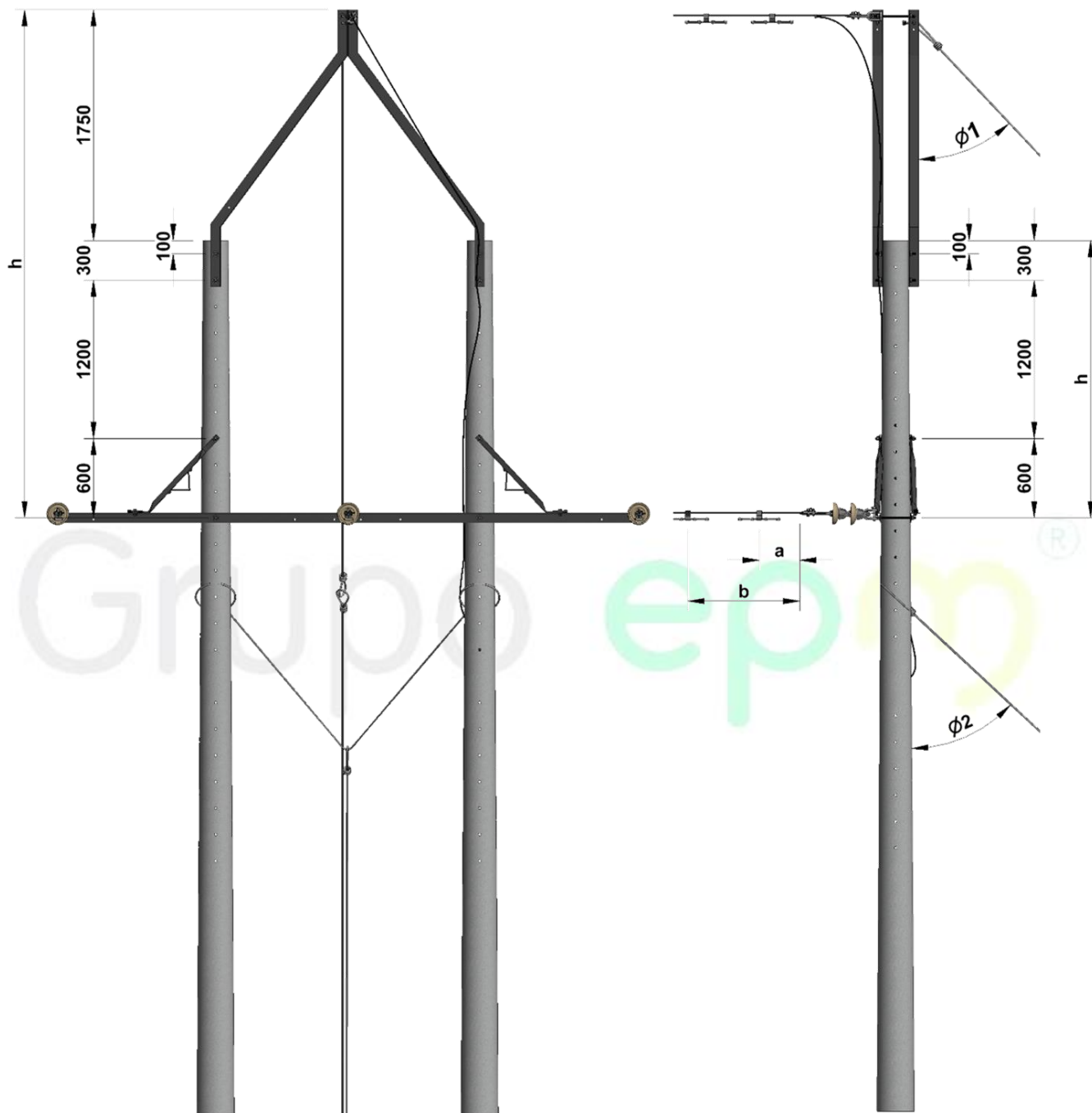
Figura 2. Vista frontal
