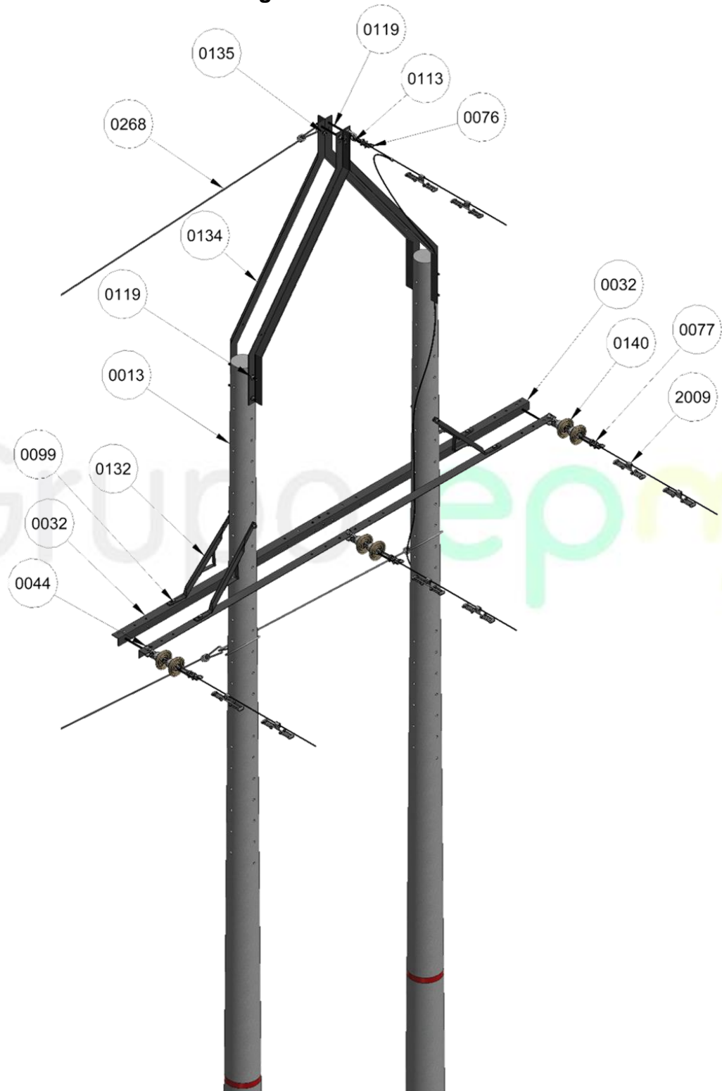
Figura 1. Vista isometrica
