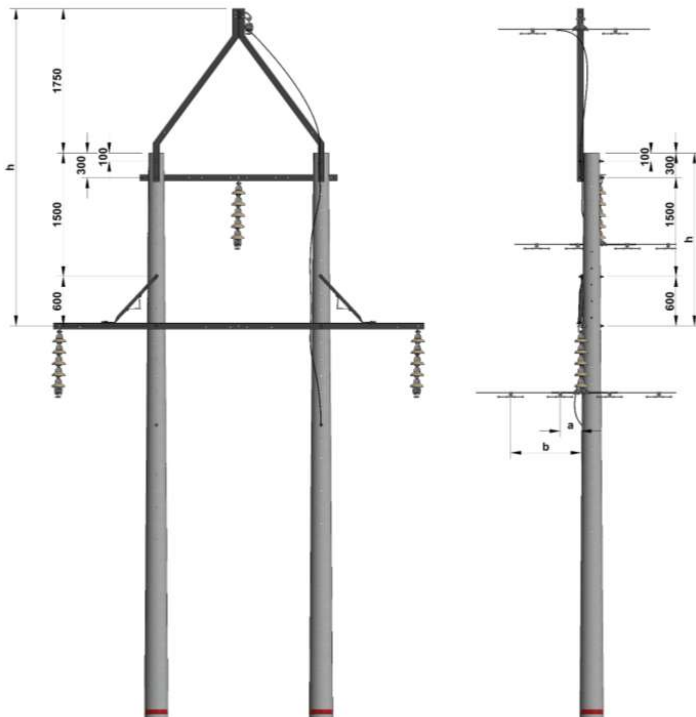
Figura 2. Vista frontal
