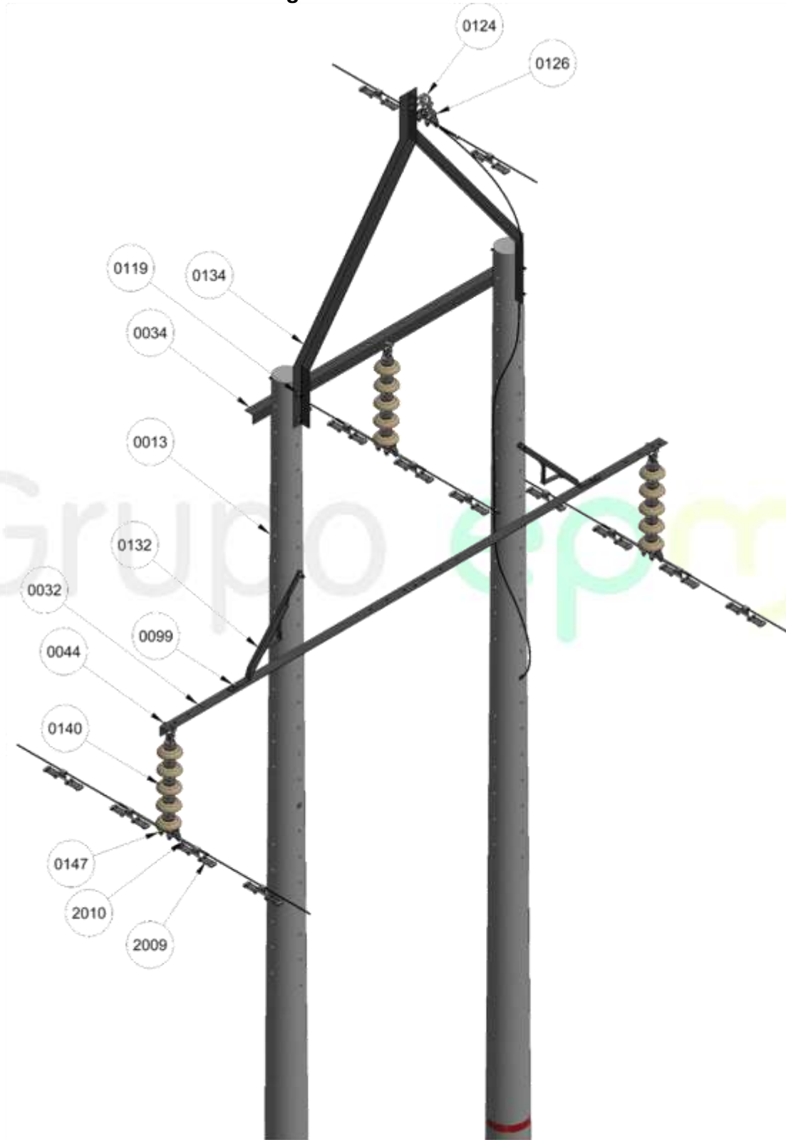
Figura 1. Vista isometrica
