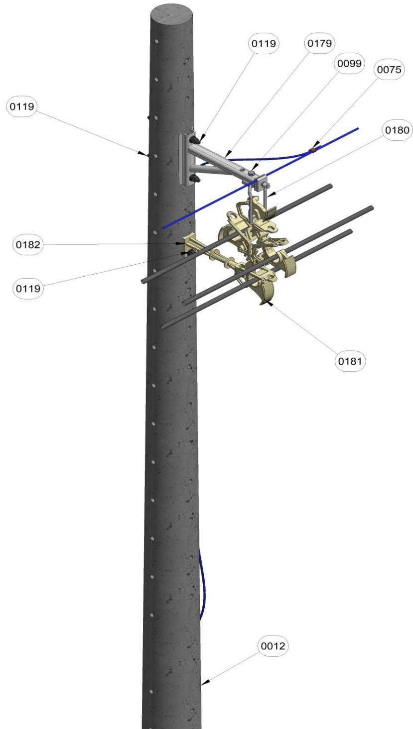
Figura 1. Vista isometrica.
