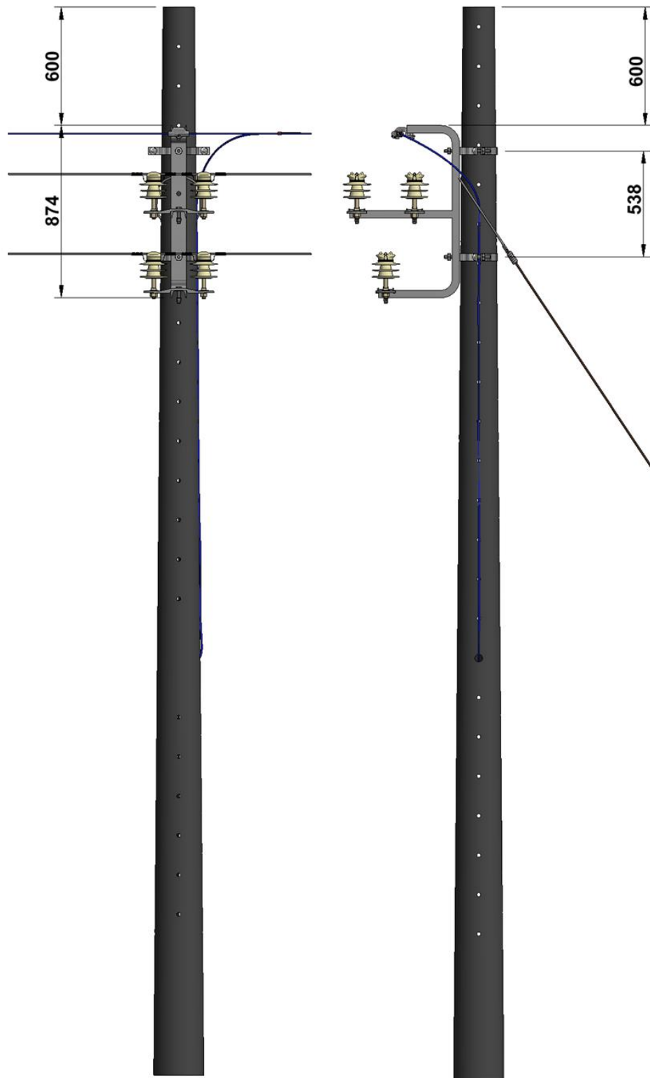
Figura 2. Vista frontal.
