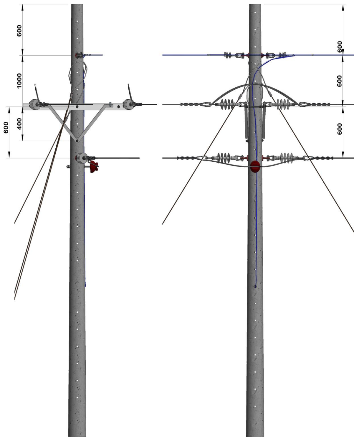
Figura 2. Vista frontal.
