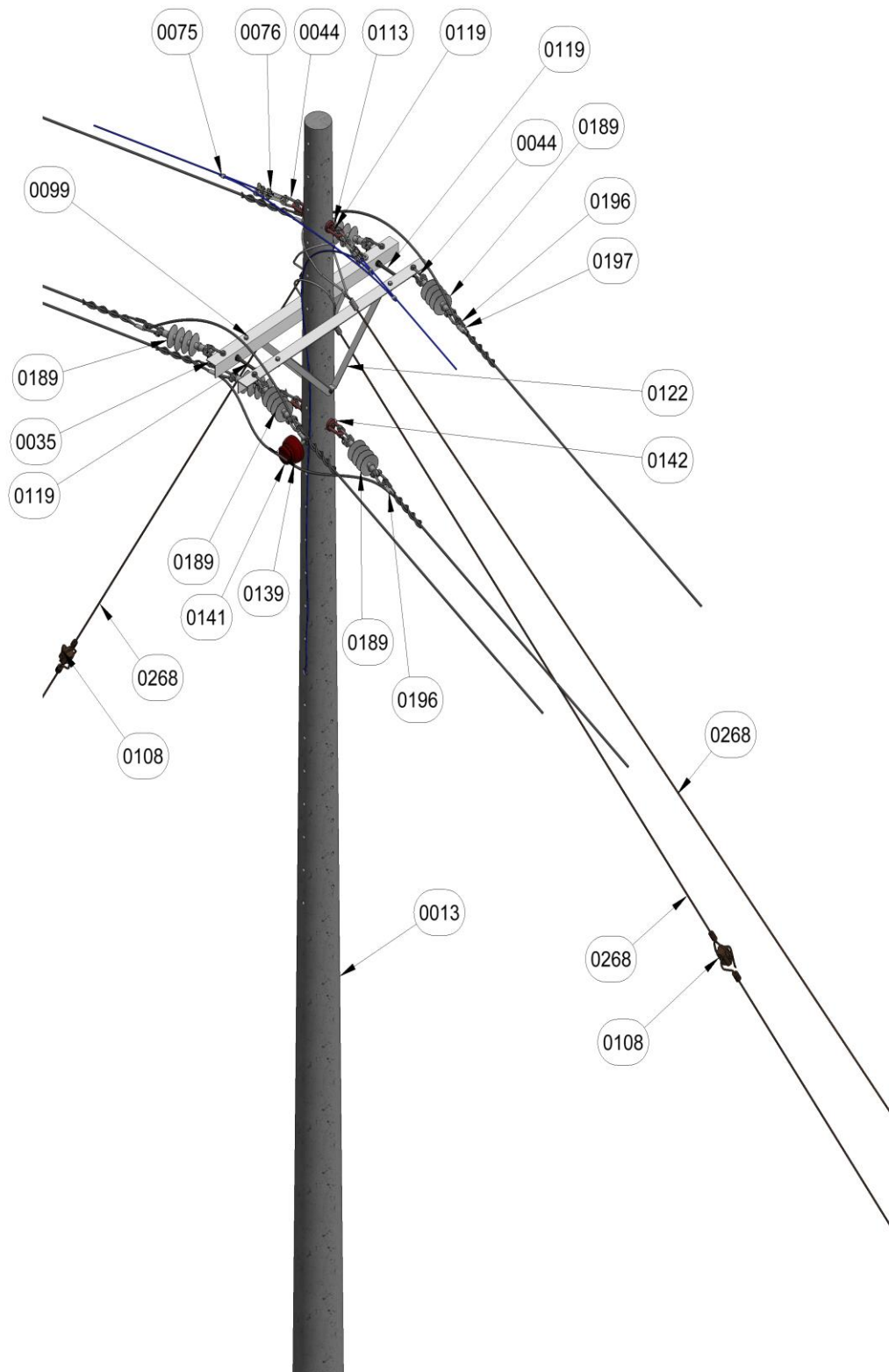
Figura 1. Vista isometrica.
