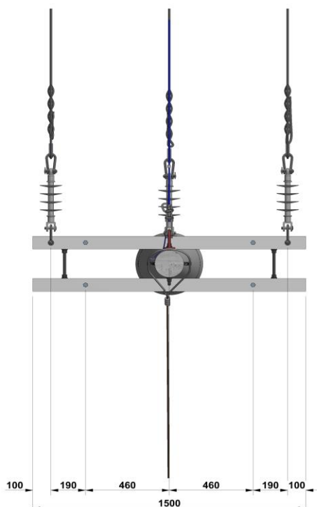
Figura 3. Vista en planta.
