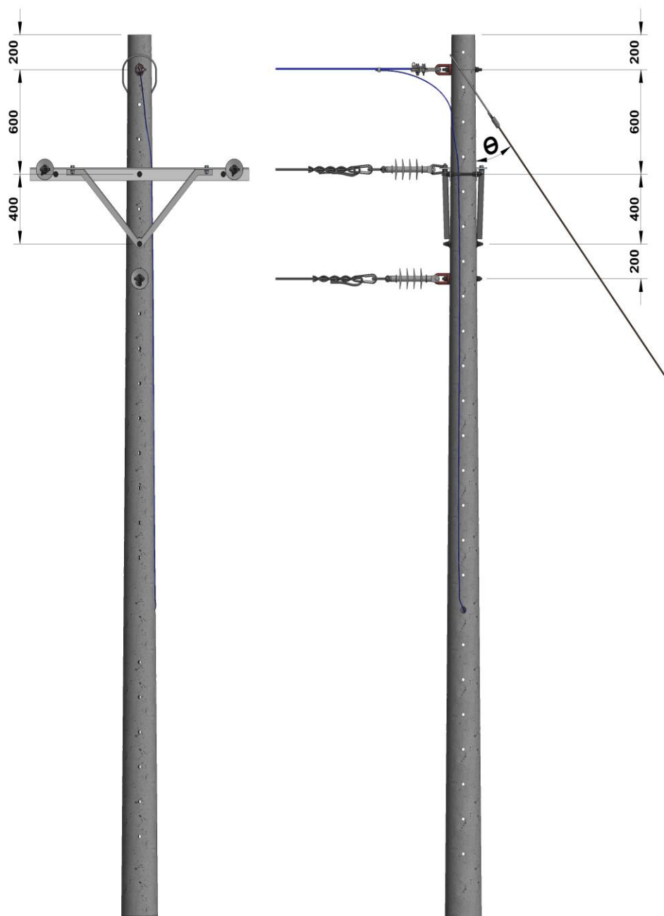
Figura 2. Vista frontal.
