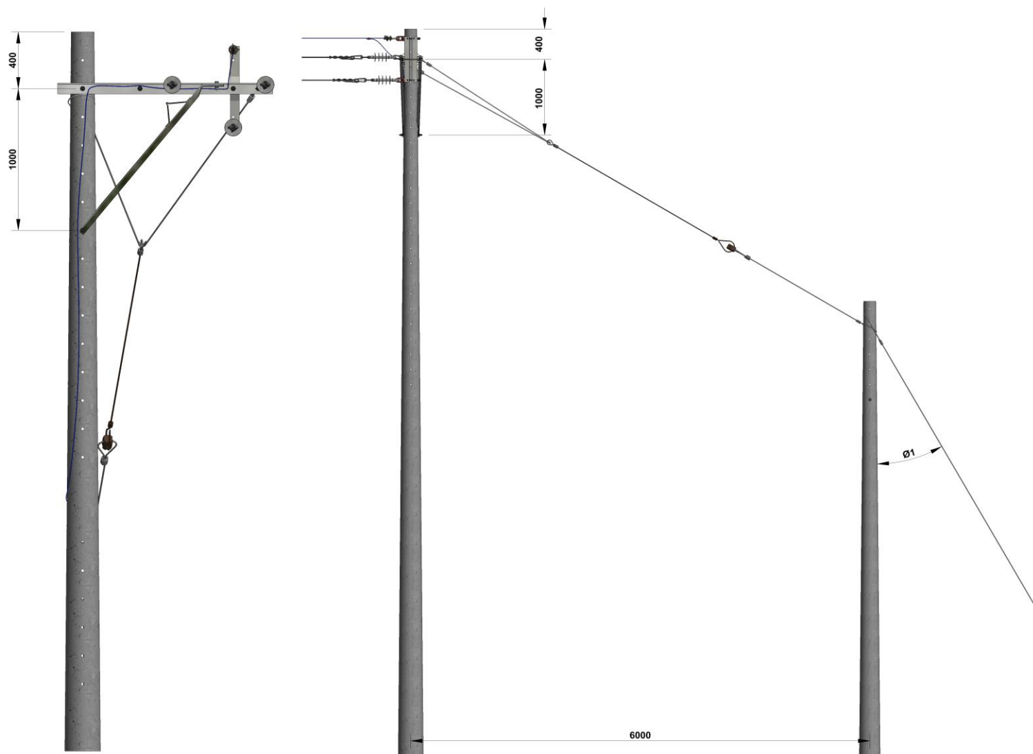
Figura 2. Vista frontal.
