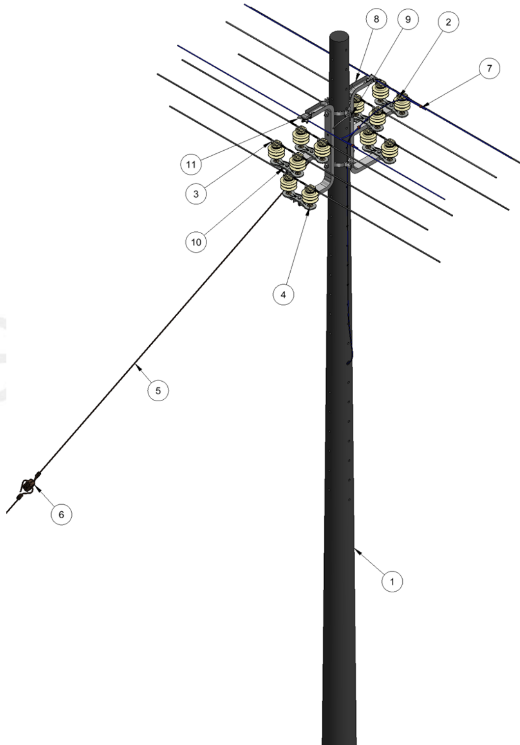
Figura 1. Vista isométrica.
