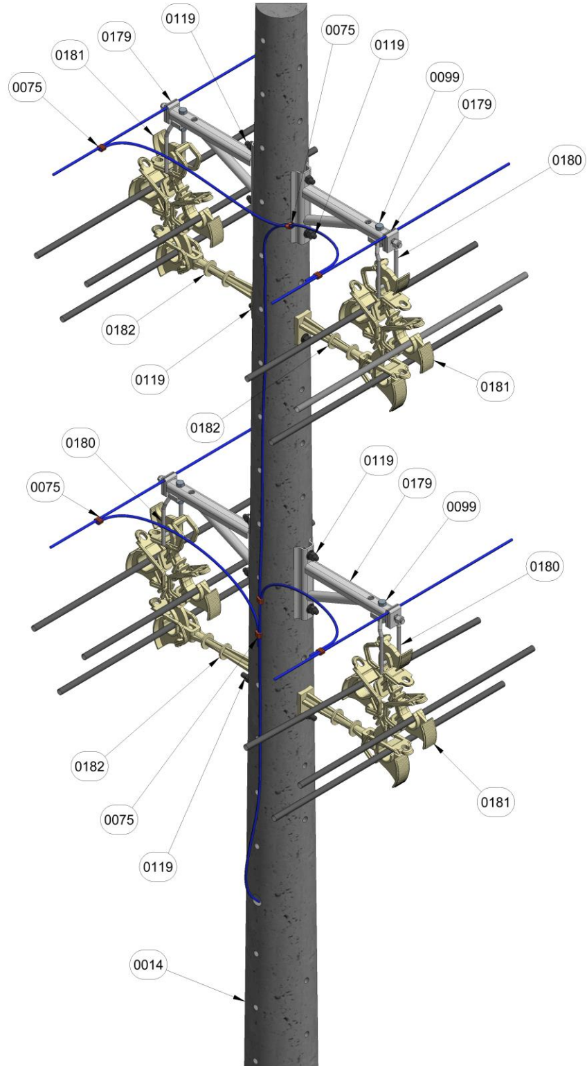
Figura 1. Vista isometrica.
