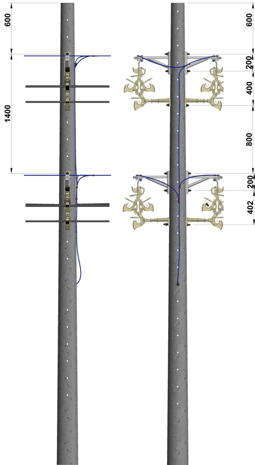
Figura 2. Vista frontal.
