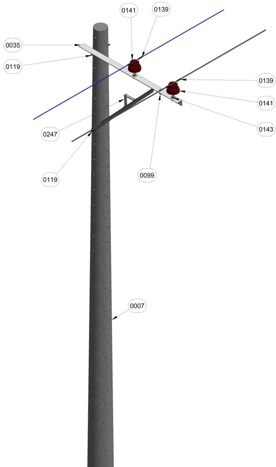
Figura 1. Vista isometrica.
