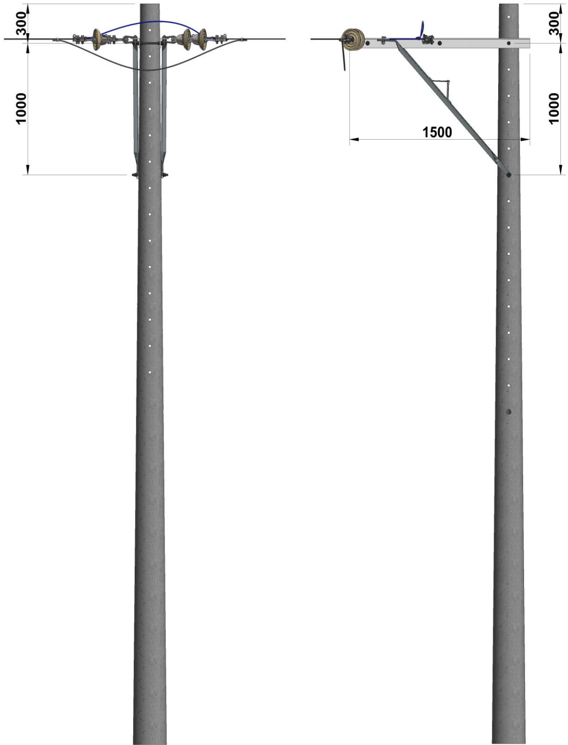
Figura 2. Vista frontal.
