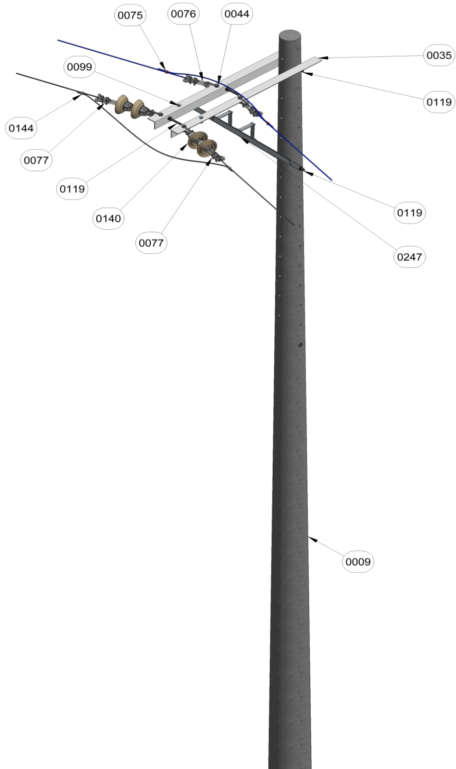
Figura 1. Vista isometrica.
