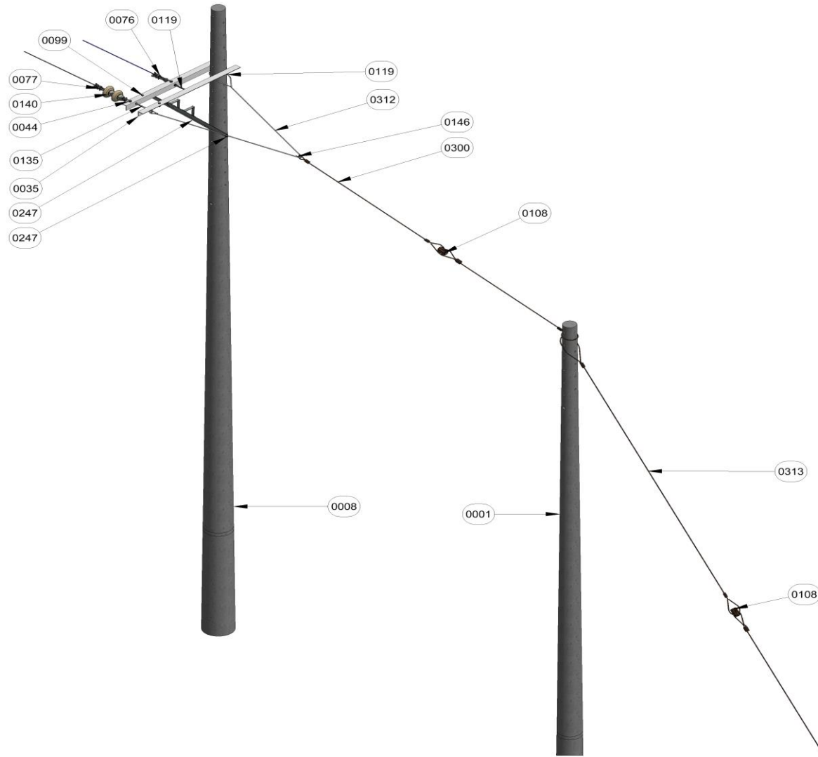
Figura 1. Vista isometrica.
