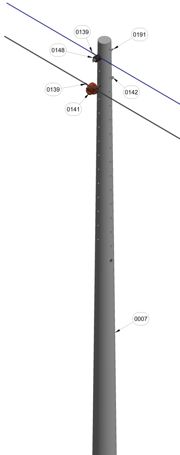
Figura 1. Vista isometrica.
