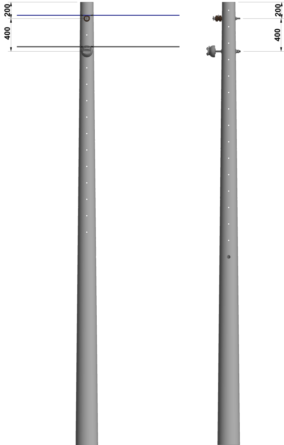
Figura 2. Vista frontal.
