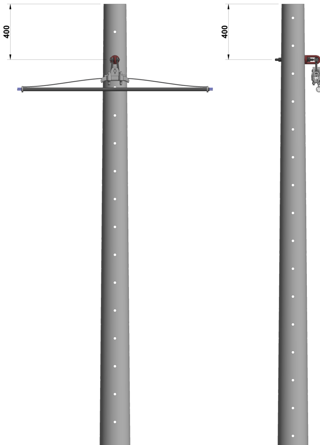
Figura 2. Vista frontal.
