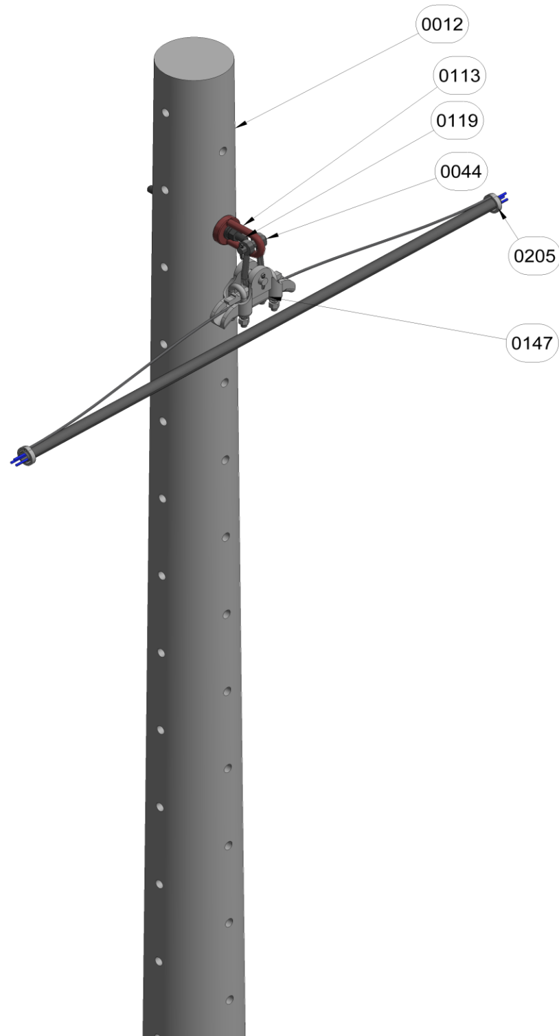
Figura 1. Vista isometrica.
