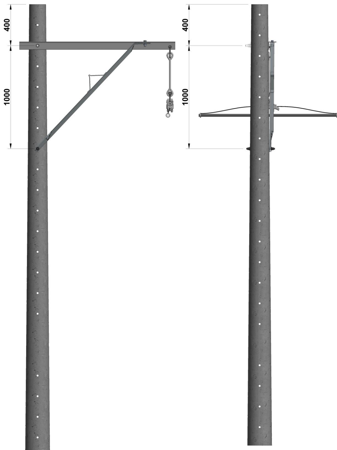
Figura 2. Vista frontal.
