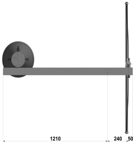
Figura 3. Vista en planta.
