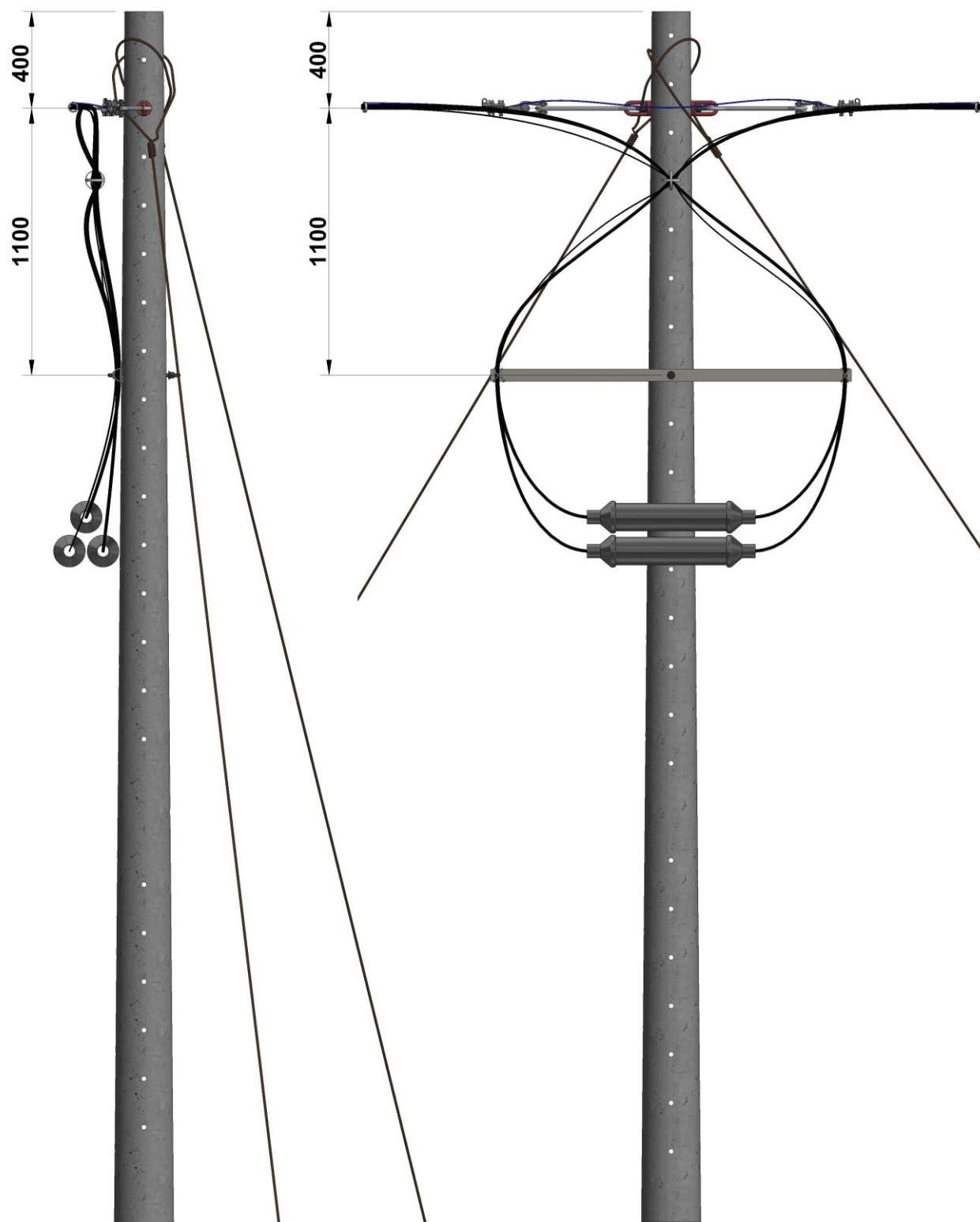
Figura 2. Vista frontal.
