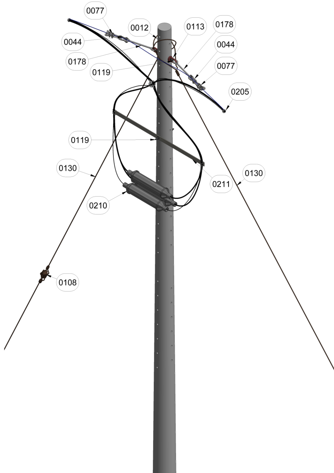
Figura 1. Vista isometrica.
