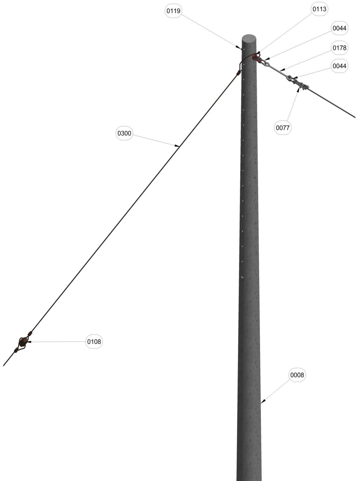
Figura 1. Vista isometrica.
