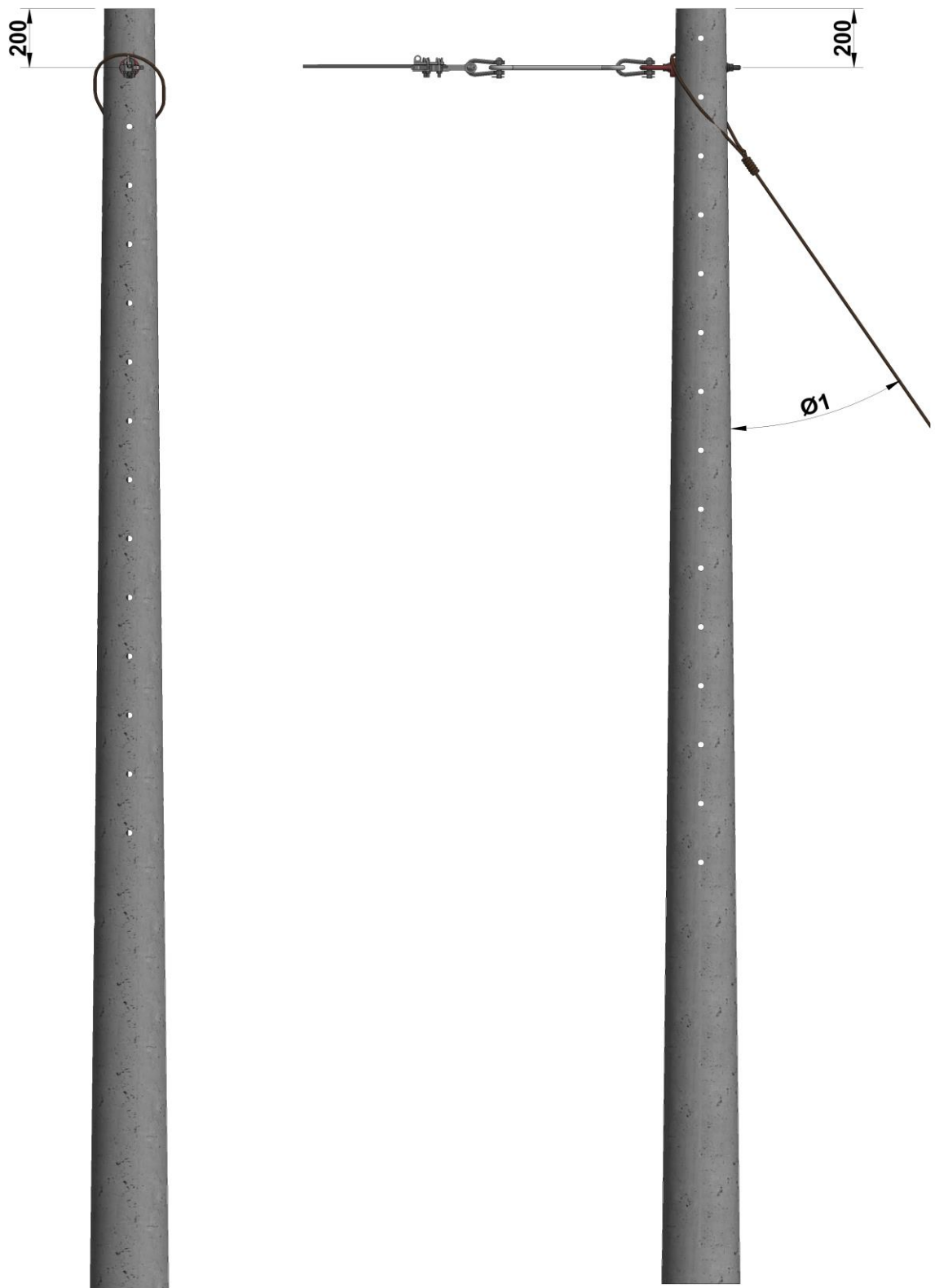
Figura 2. Vista frontal.
