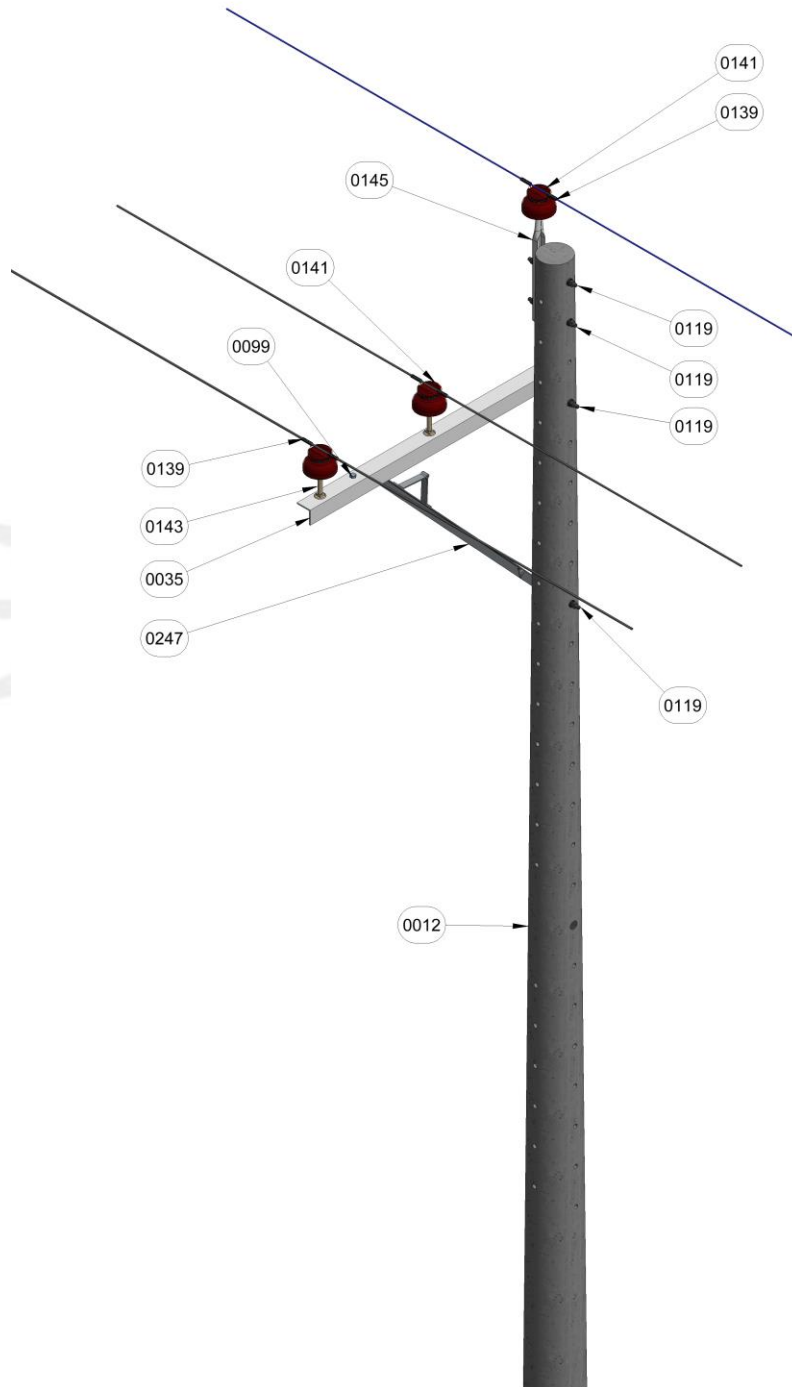
Figura 1. Vista isometrica.
