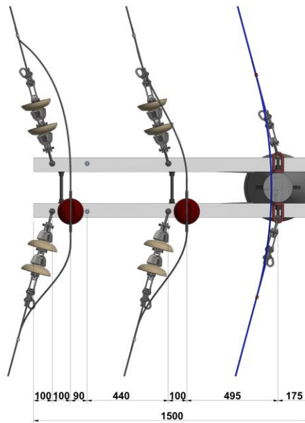
Figura 3. Vista en planta.
