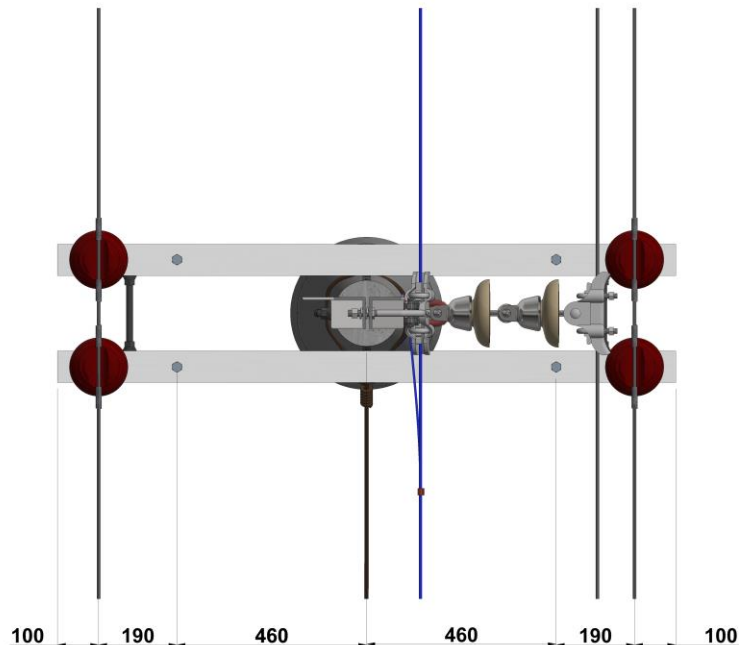
Figura 3. Vista en planta.
