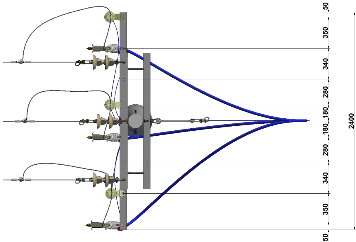
Figura 3. Vista en planta.
