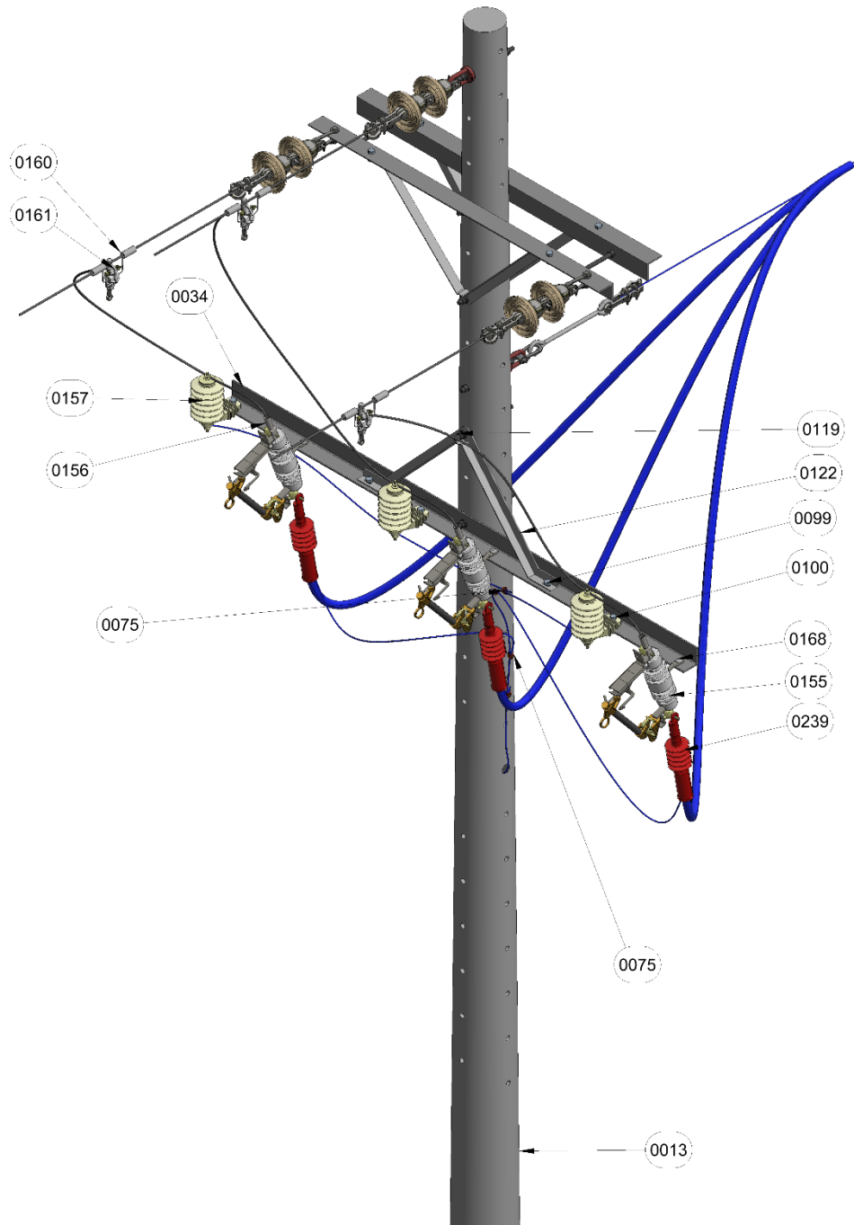
Figura 1. Vista isometrica.
