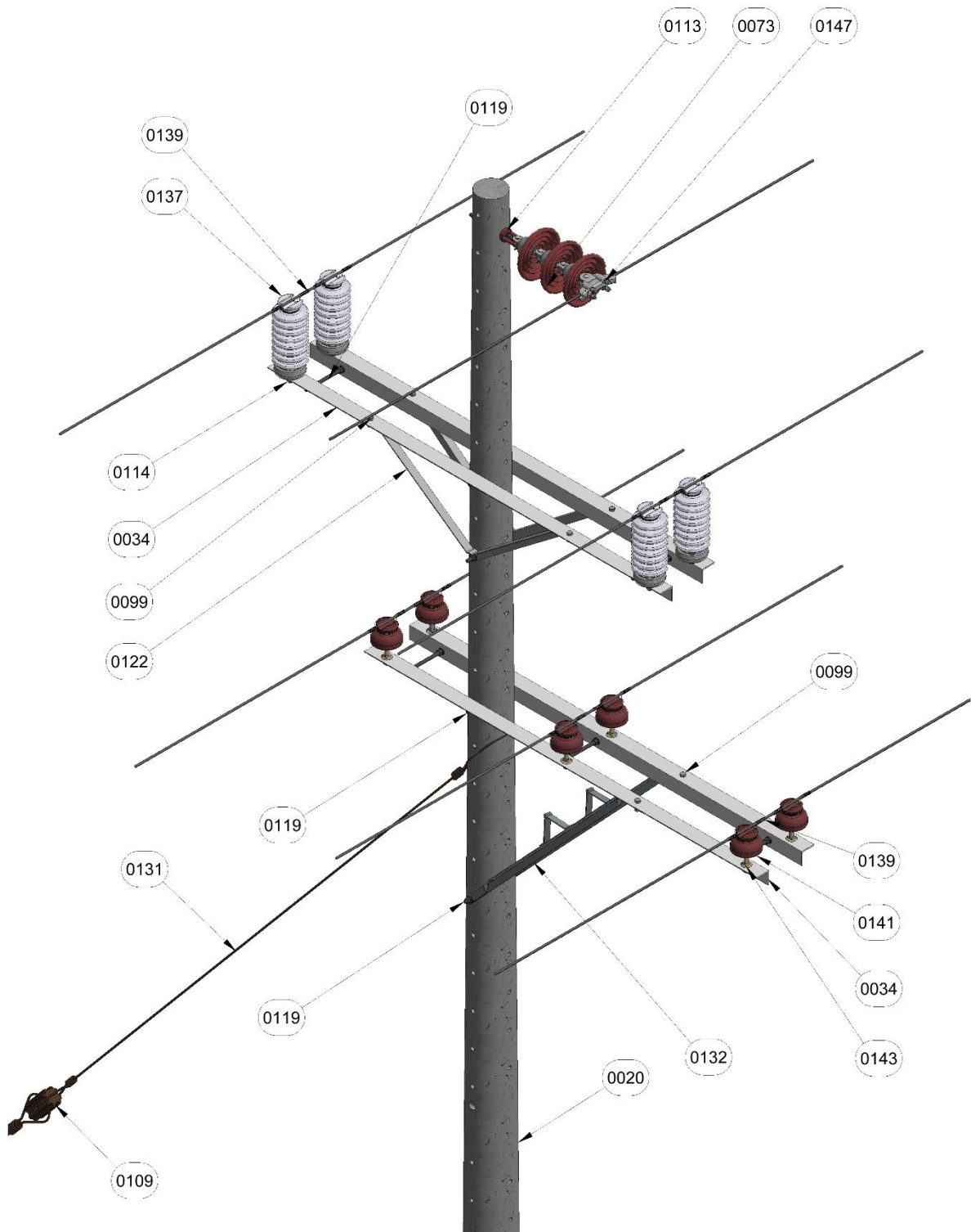
Figura 1. Vista isometrica.
