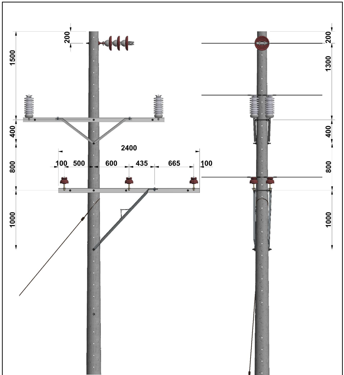
Figura 2. Vista frontal.
