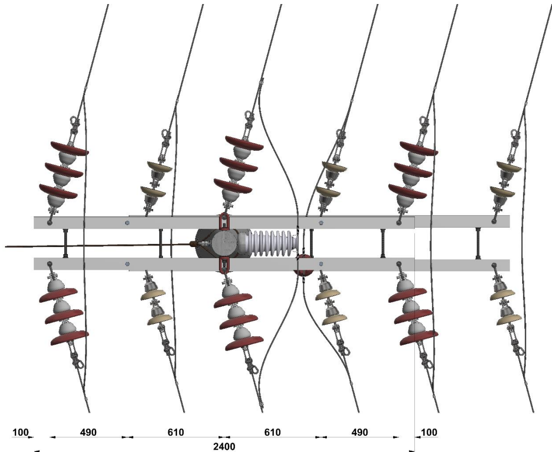
Figura 3. Vista en planta.
