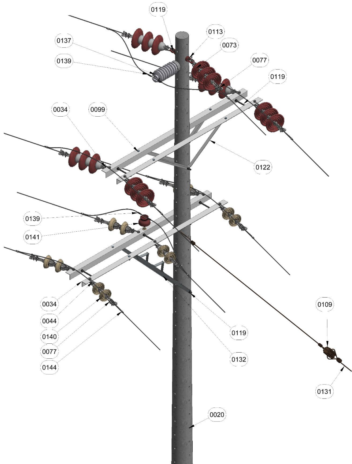
Figura 1. Vista isometrica.
